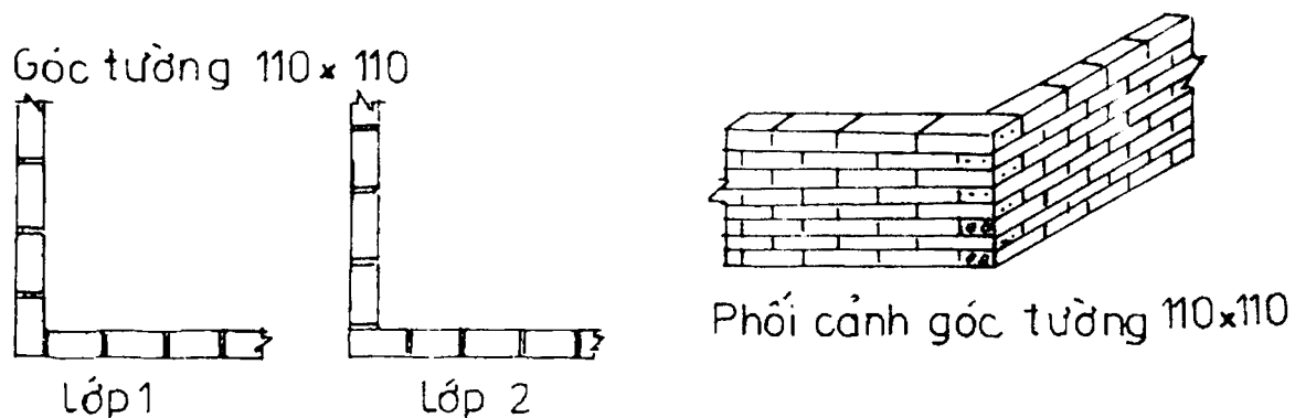
Hình 4.1: Cấu tạo góc tường 110 (tường con kiến)
