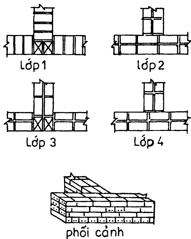
Hình 4.3: Cấu tạo tường chữ đinh 220 (T)
