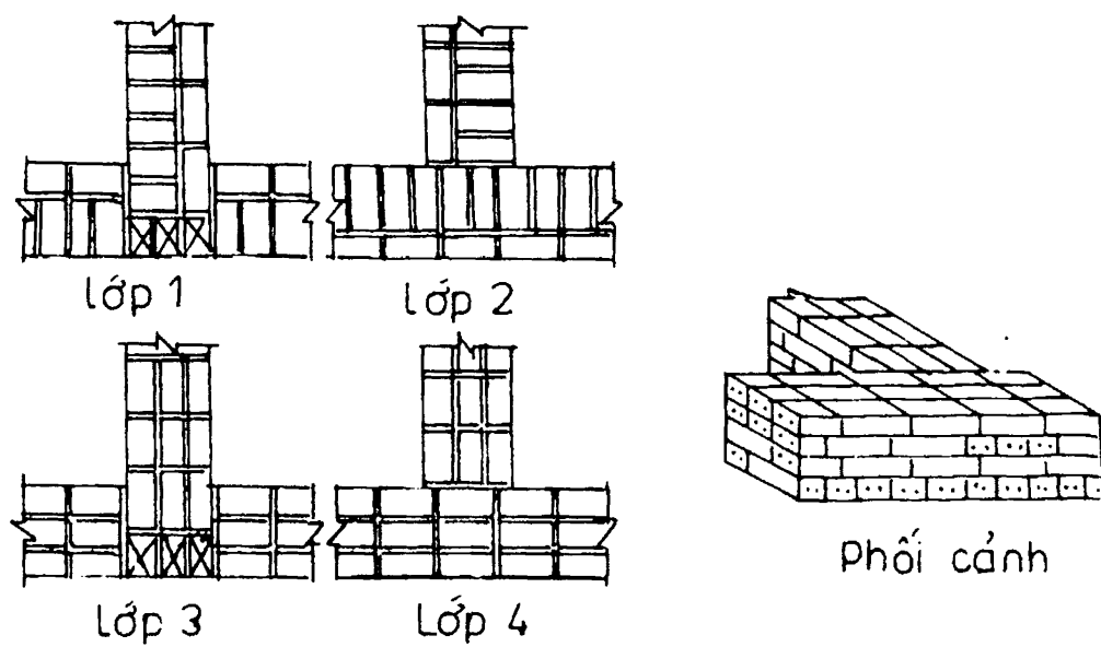
Hình 4.6: Cấu tạo tường chữ đinh 330 (┐)
