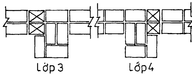
Hình 4.8: Cấu tạo trụ liên tường (trụ 220 \times 220 tường 110; trụ 330 \times 330 tường 220; trụ 330 \times 450 tường 220)
