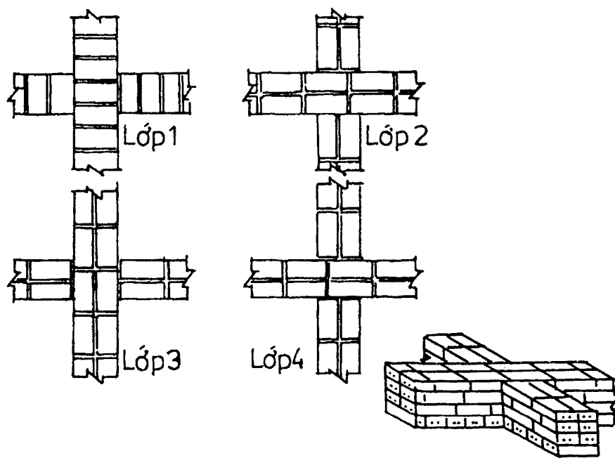
Hình 4.4: Cấu tạo tường chữ thập 220 (+)
