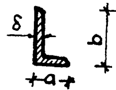
Bảng 3.10 Quy cách thép góc không đều cạnh L [43]
