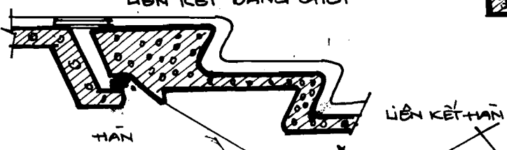
H. 37a. LIÊN KẾT GIỮA CÁC CẦU KIÊN LIÊN KẾT BẰNG CHỐT
