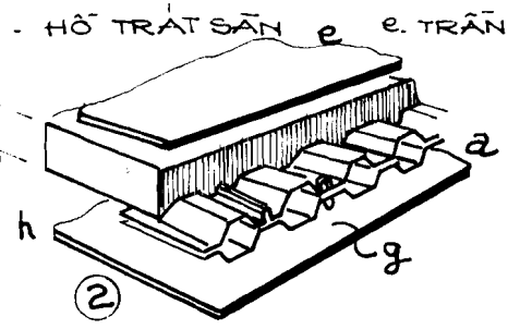
H.4.28: SÀN DÂY TÔN THÉP ĐỊNH HÌNH
