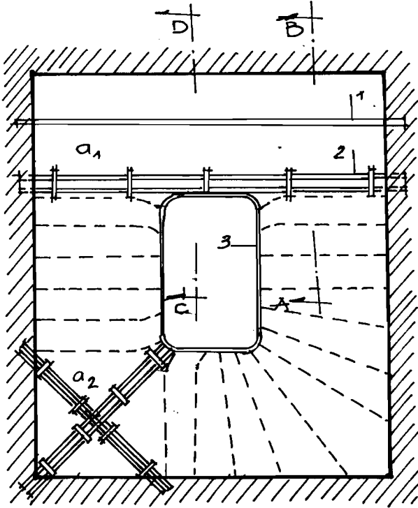
H6.25 LIÊN KẾT DÂY THANG VÀO DÂY CHÌU NGHĨ
