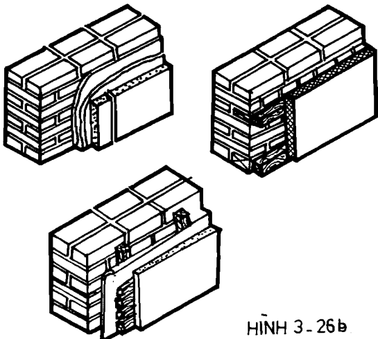
TƯỜNG GIỮ NHIỆT VÃ CÁCH NHIỆT TƯỜNG NHIỀU LỚP
