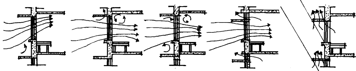
Hình 3-12 TẤM CHE CHẮN NẮNG
