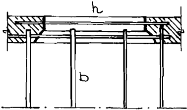
H.4.17: BỐ TRÍ DÂY SÀN THÉP
