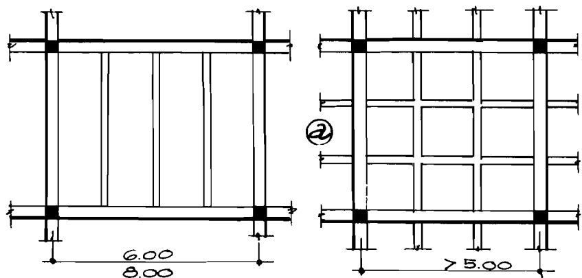
H. 4-32 SÀN B.T.C.T Ô CỜ (a) Ô VUÔNG (b) Ô QUÁ TRÀM
