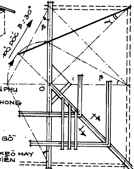
H 7-212 KHU NÓC TIẾT DIỆN NGANG CẦU PHONG VÀ THANH KÈO CHỊU MĂNG XÔI VÀ GỖ SÔNG NÓC
