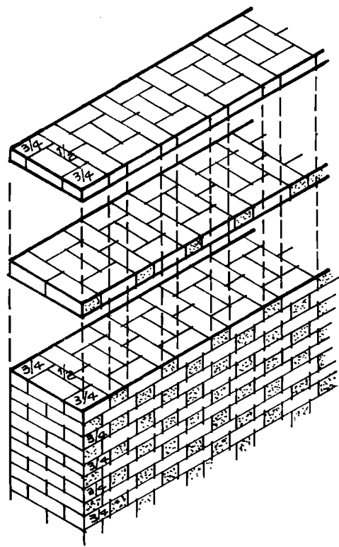
H3.2d TƯỜNG 2 GẠCH
