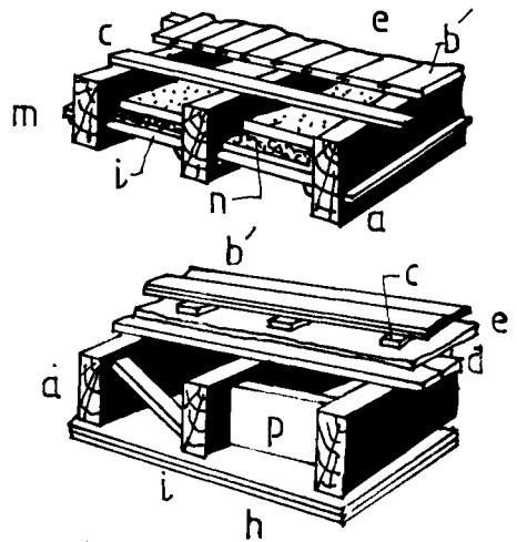
SÀN GỖ CÁCH NHIỆT - ÂM
