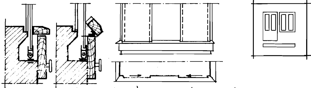
H.5.31 CỬA BẰNG KÍNH - CHẤT Dẻo - CHI TIẾT HẦM ỔN ĐỊNH
