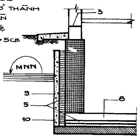
(d) LỚP CÁCH NƯỚC Ở PHÍA NGOÀI
