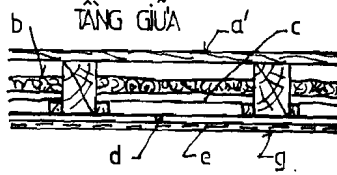
HÌNH 4.13 TRẦN TRÁT
