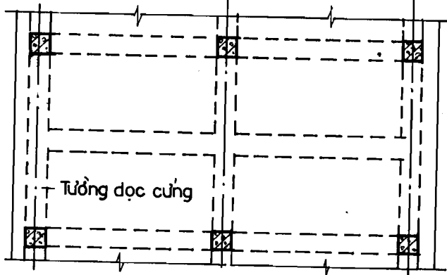
MÓNG KIỂU HỘP
