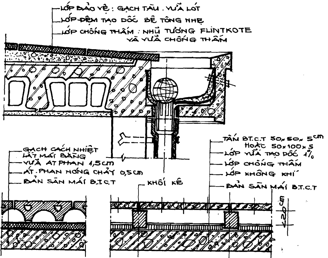
Hình 7-34 : CẤU TẠO CHÔNG THÂM VÀ ĐẢO VỆ CHÔNG THÂM MÁI BĂNG
