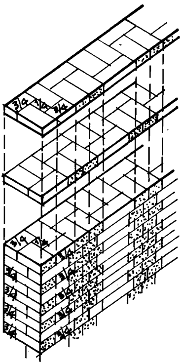
H3.2C TƯỜNG MỘT GẠCH RỬỚI
