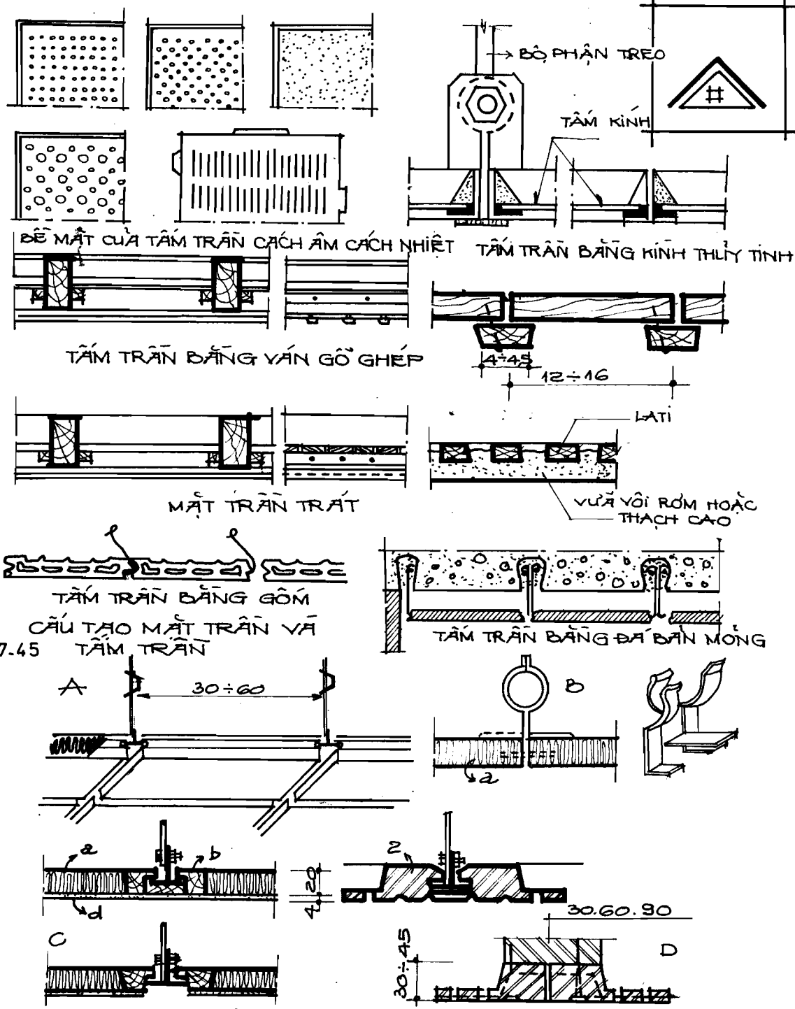
Hình. 7-46 CHI TIẾT TREO TẦM TRẦN
