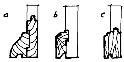
HÌNH 5.25 B CHI TIẾT CẤU TẠO GỖ MŨI NƯỚC a. GỖ MŨI NƯỚC BẰNG GỖ LIÊN KẾT VỚI KHUNG CỬA ĐI b. CẤU TẠO CHI TIẾT GỖ MŨI NƯỚC CHO CỬA c. KHUNG CỬA KẾT HỢP GỖ MŨI NƯỚC CHO CỬA
