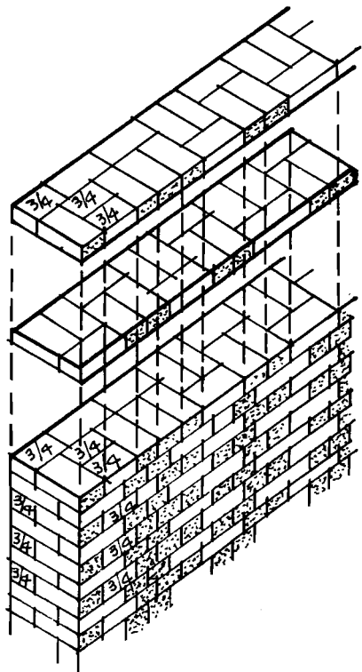
H3.2C TƯỜNG MỘT GẠCH RỬỚI
