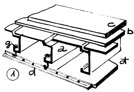
H.4.28: SÀN DÂY TÔN THÉP ĐỊNH HÌNH
