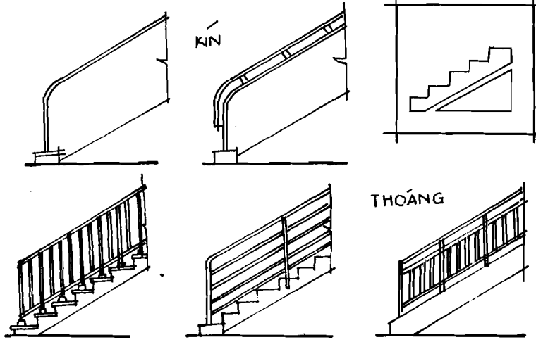
HINH 6 - 38 LAN CAN - TAY VIN
