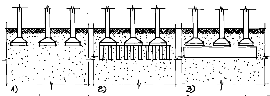
Hình 2.5b CÁC LOẠI MÓNG NHÀ TƯỜNG KHỐI KHI ĐẤT YẾU (RỐI) 1) KHI TẢI TRỌNG NHỎ. 2,3) KHI TẢI TRỌNG TRUNG BÌNH.
