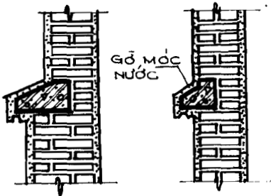
H.3.17 BÊ TƯỜNG
