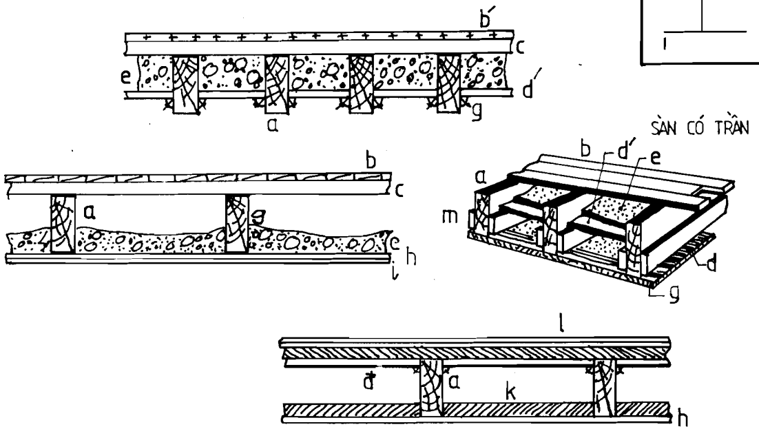
SÀN CÓ TRẦN - DÂM LỘ
