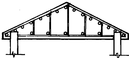
Hình 7.42A TRẦN TREO
