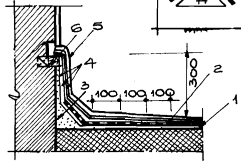
CHỐNG THẨM BẰNG GIẤY DẦU (Hình 7.33A)
