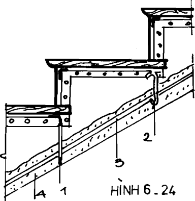
SƯỜN TRẦN LIÊN KẾT TREO BẰNG THÉP TRÒN HOẶC THÉP ĐÀN VÀO SƯỜN ĐẮC THANG
