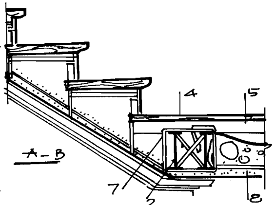
H6.25 LIÊN KẾT DÂY THANG VÀO DÂY CHÌU NGHĨ
