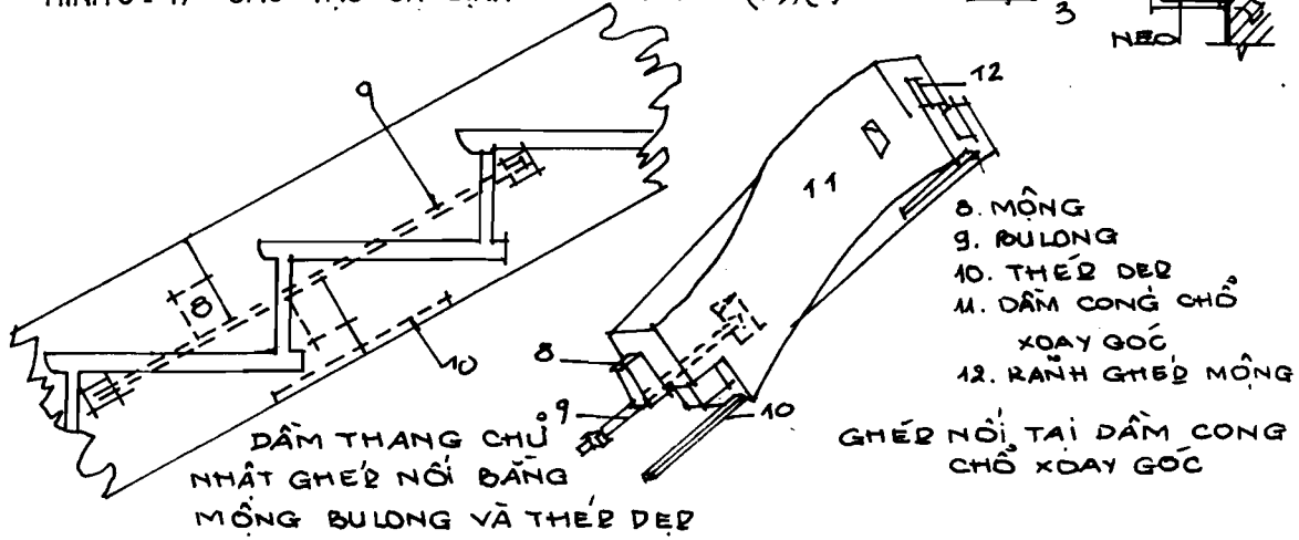
HÌNH 6-18 GHEP NỐI DẪM THANG
