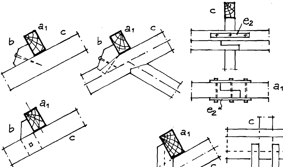
HÌNH 7.12C: LIÊN KẾT MẶT TRUNG GIAN.
