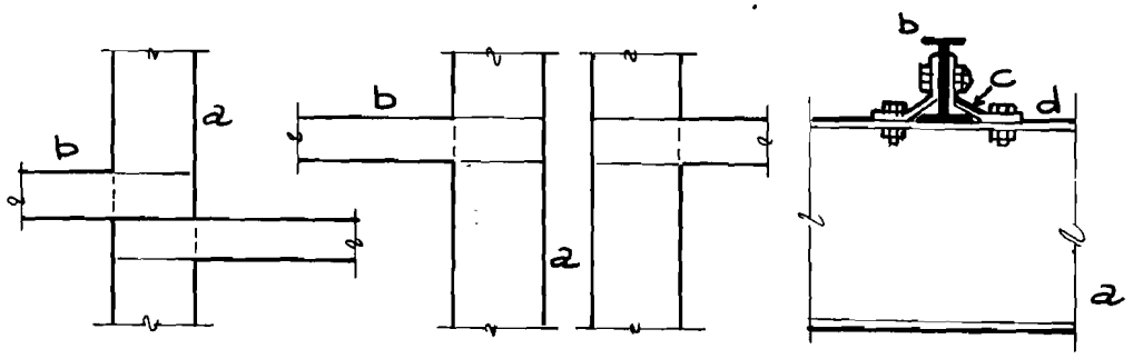
H.4.21: DÃM PHỤ GÁC LÊN DÃM CHÍNH
