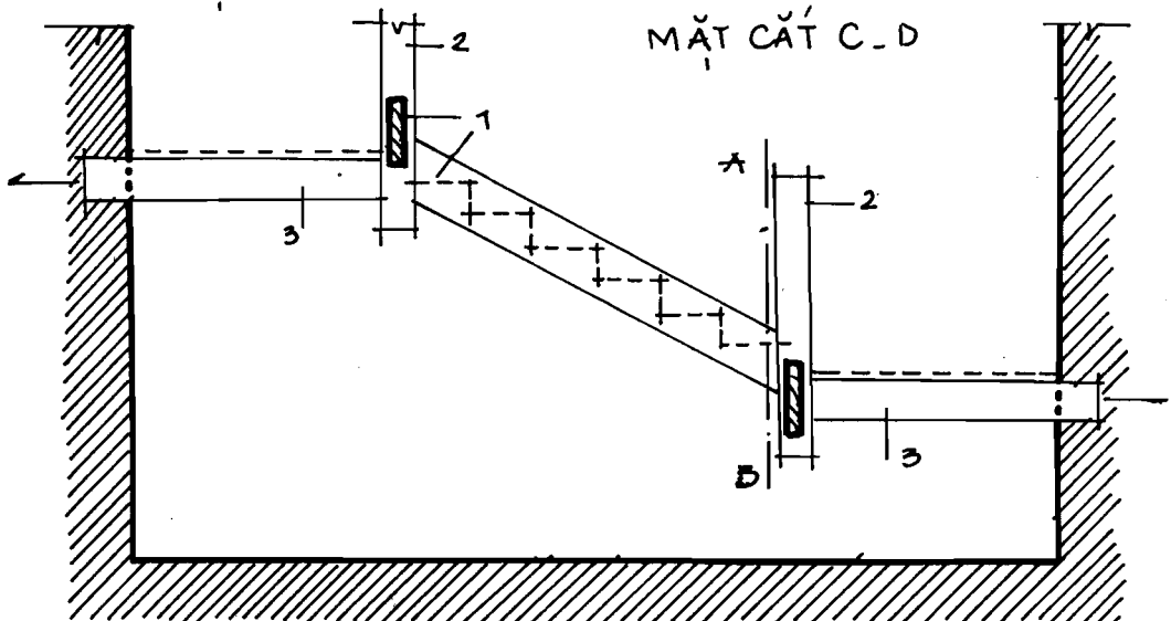
HÌNH 6-19b CẤU TẠO CHIỀU NGHI GIẢI THÁP DẦM THANG VÀ TRỤ ĐỤY TRUNG GIÀN.
