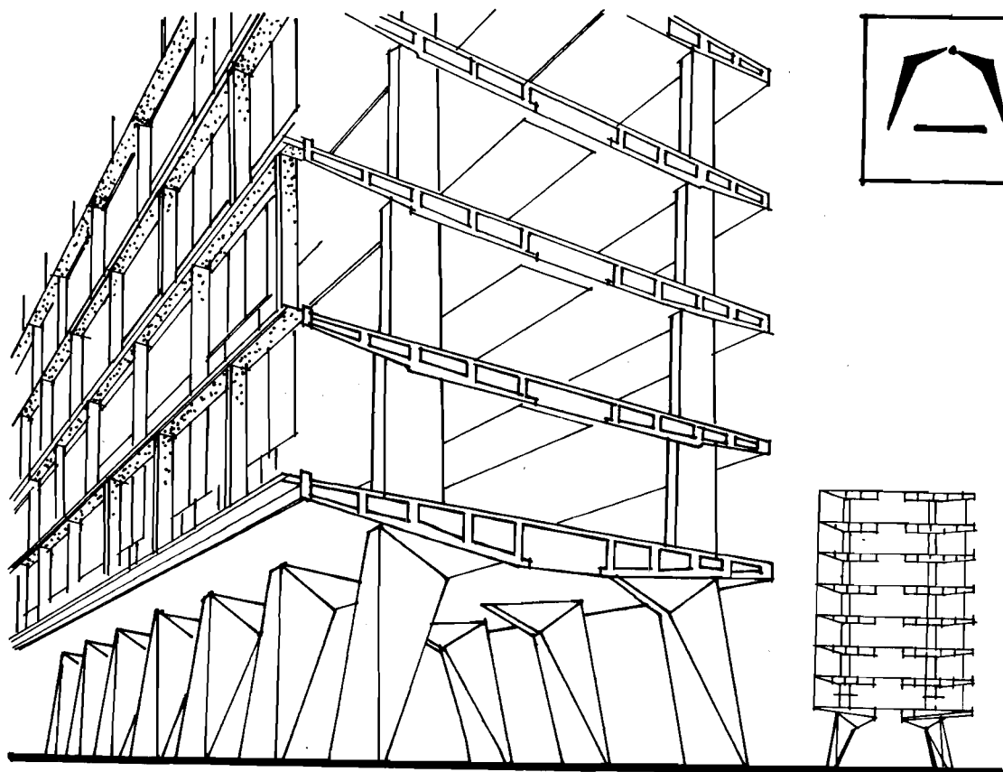
H 1.4 KẾT CẤU KHUNG HOÀN TOÀN
