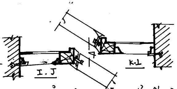
HÌNH 6-19a CẤU TẠO CHIỀU NGHI', GIẢI PHÁP dầm chiều nghi' chịu lực chính
