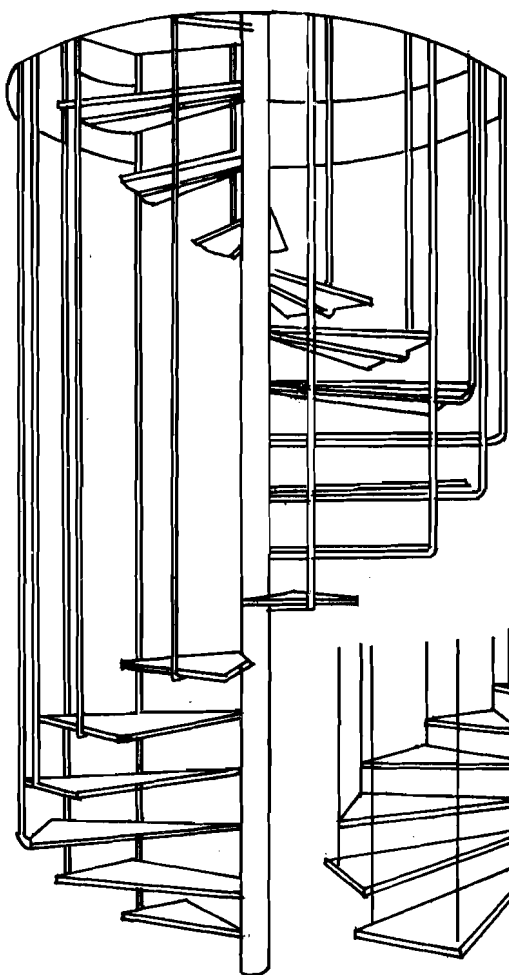
H6_40a_ Cầu thang tròn xoay trên ốc
