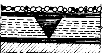
f. 1. ĐÁ SẠN 2. BI TUM 3. LỚP CHỐNG THẨM 4. KẾT CẤU CHỊU LỰC
