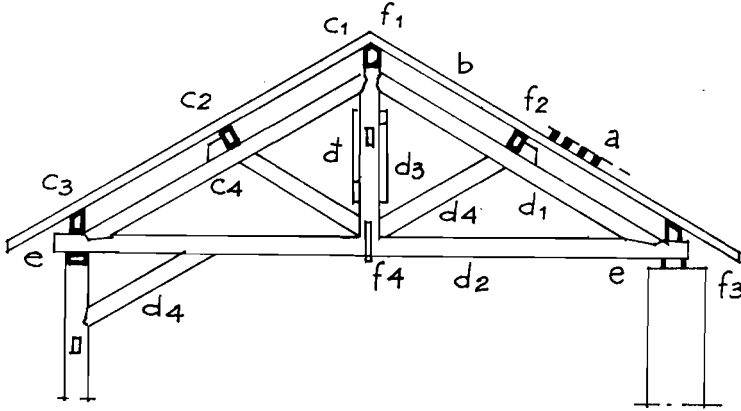
HÌNH 7.11 MÔ TẢ CẤU KIỆN 1 SƯỜN NÓC VỚI DÀN VỊ KÈO GỖ
