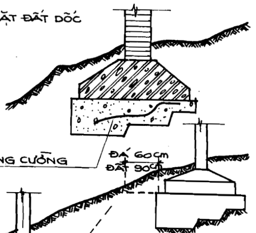
MÓNG CHIẾC DƯỚI CỘT
