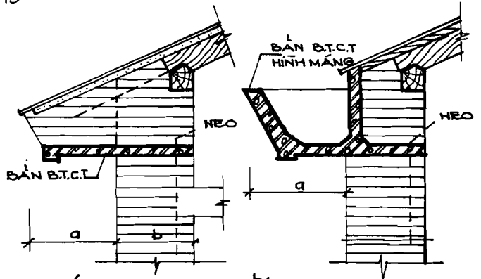
MÁI ĐUA KHI a > b/2
