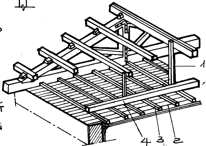
Hình 7.42A TRẦN TREO
