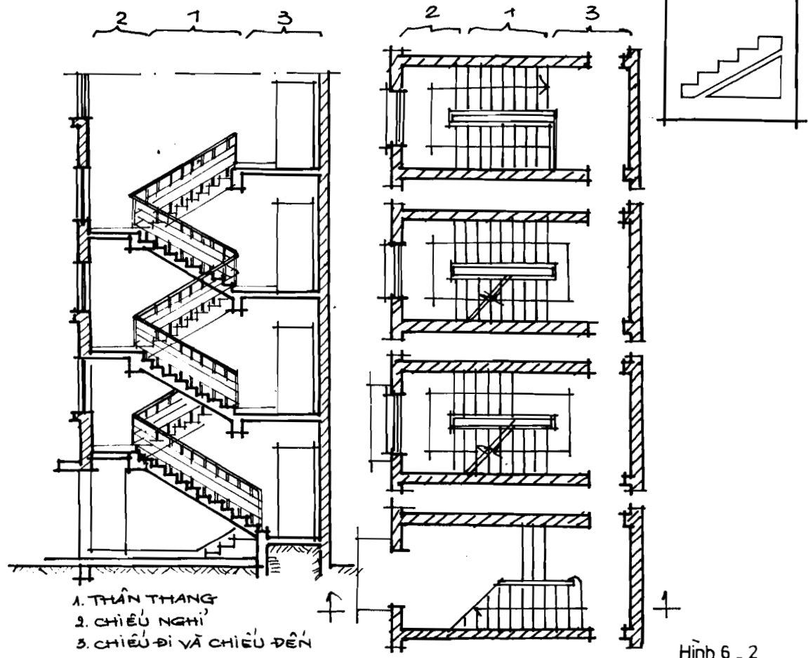
CÁC BỘ PHẬN CƠ BẢN CỦA CẦU THANG (M. BÃNG & CẮT)
