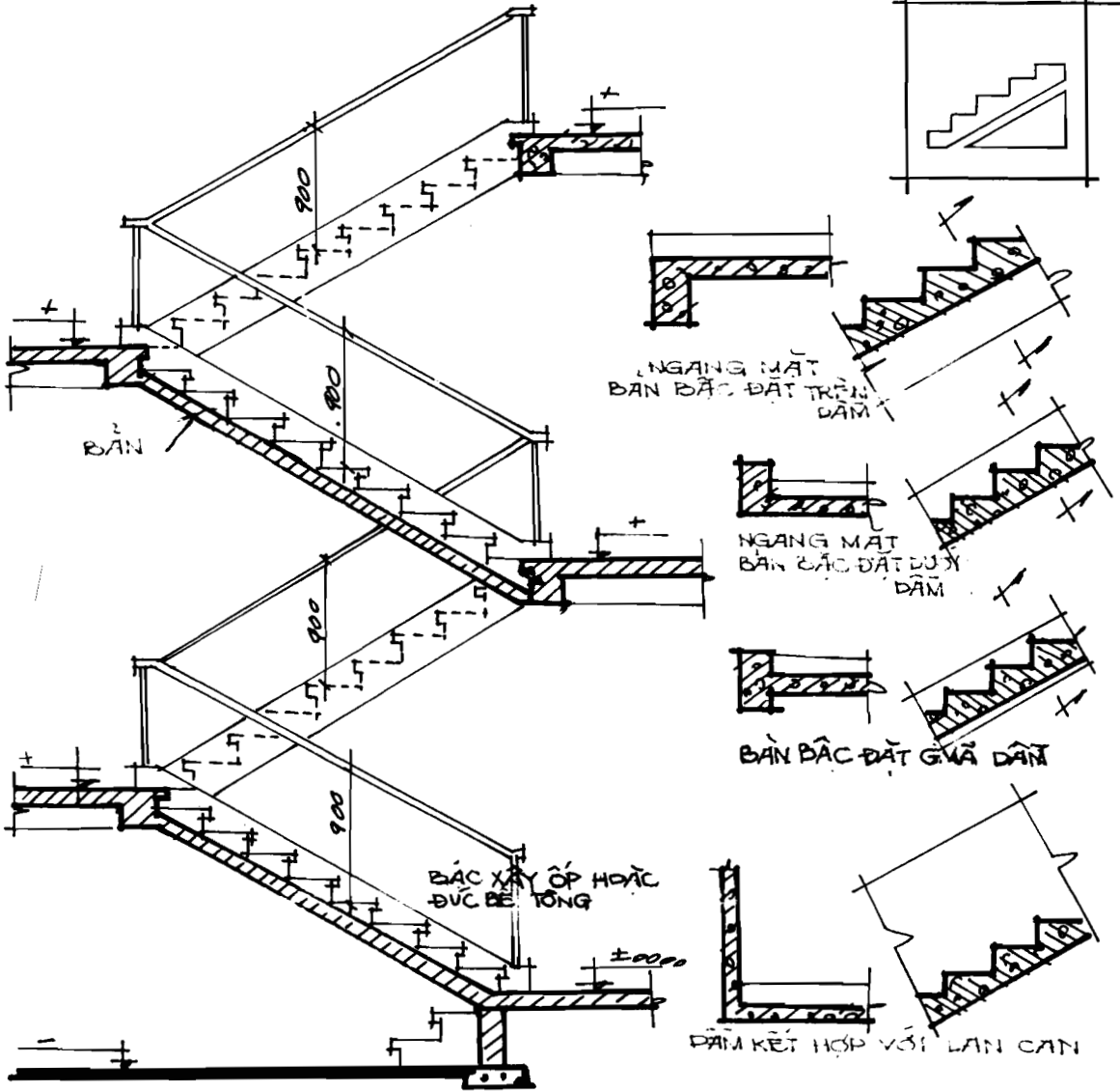
H6.32 b . CẦU THANG B.T.C.T TOÀN KHỐI HÌNH THỨC BẢN DẦM
