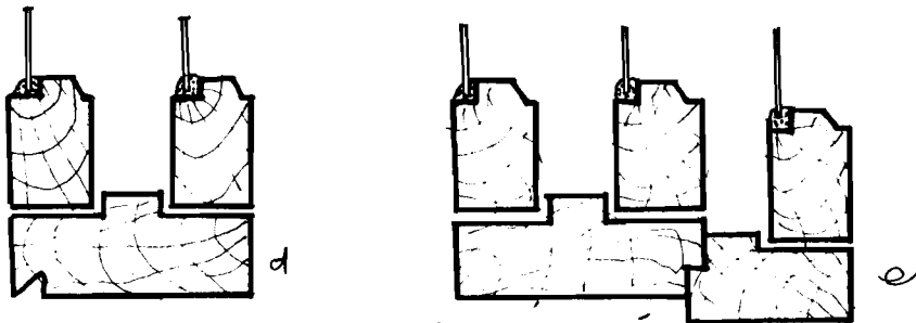
Hình 5-16B: CẤU TẠO CỬA NHIỀU LỚP
