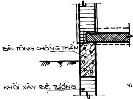
H.3.17 BÊ TƯỜNG
