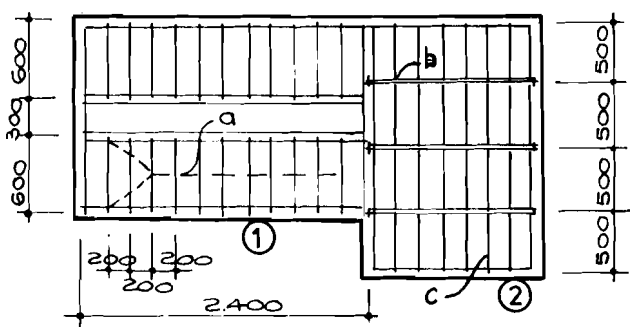
H.4.18: SƠ ĐỒ BỐ TRÍ DÂY SÀN SẮT THÉP
