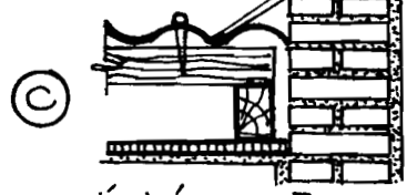
c. MŨ GIÁP NHÀ VÀ TƯỜNG ĐẦU HỒI
