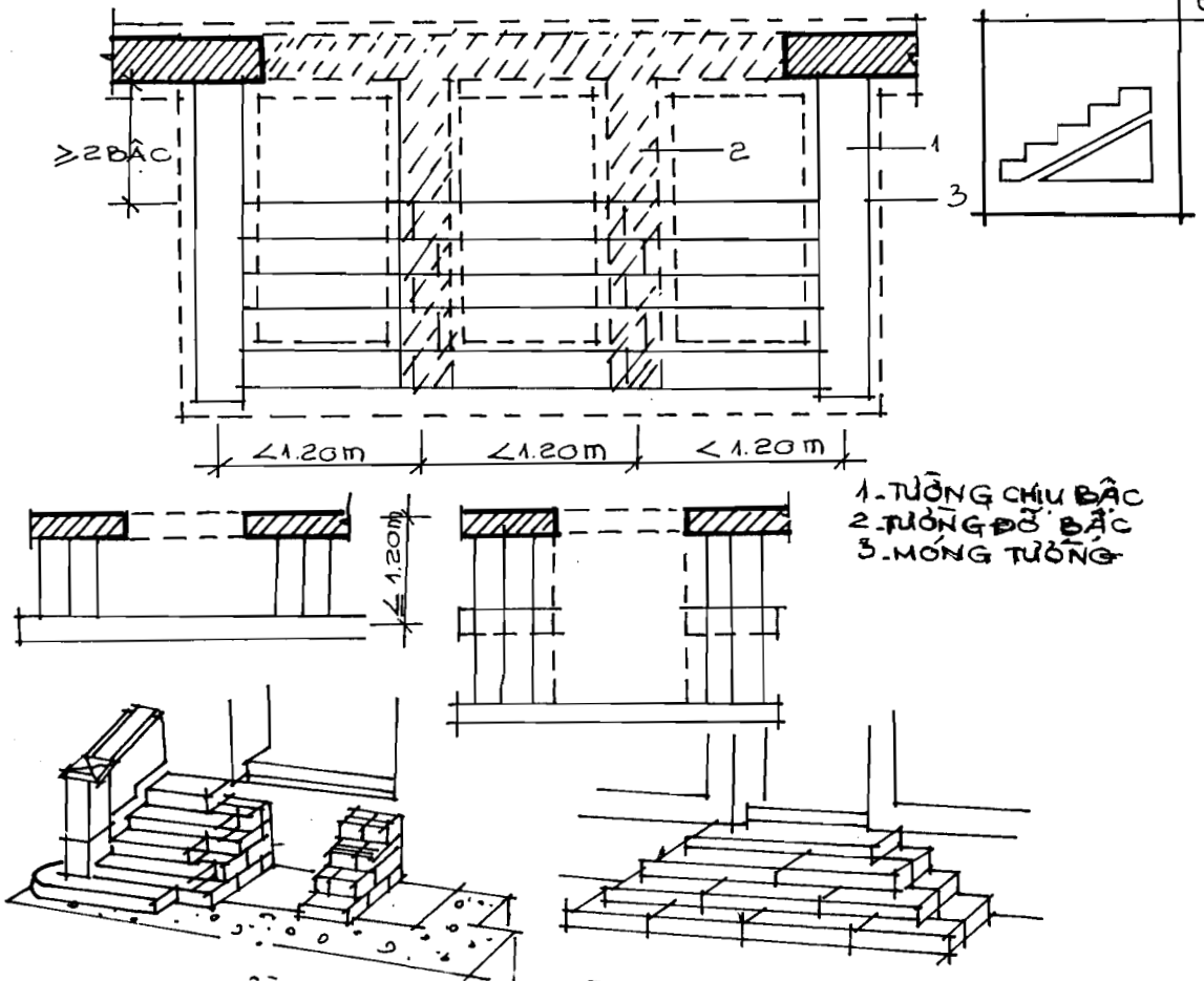
H6-29 . CẦU THANG NGOÀI NHÀ XÂY BẰNG ĐÁ
