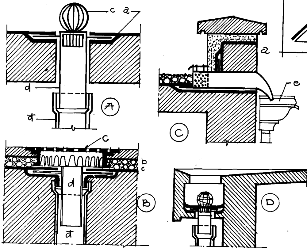
Hình 7-37 CẤU TẠO MIẾNG THU NƯỚC
