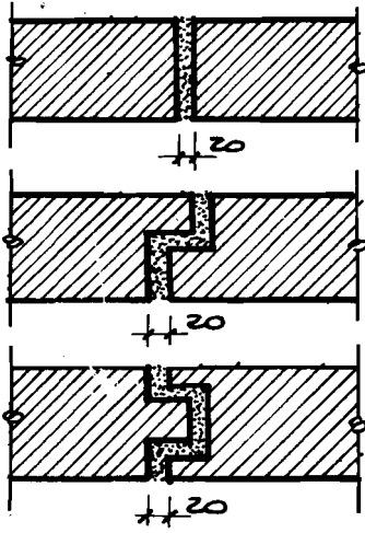
H 8.19 KHE BIẾN DẠNG
