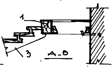
HÌNH 6-19a CẤU TẠO CHIẾU NGHỈ GIẢI THÍCH DẪM CHIẾU NGHỈ CHỊU LỰC CHÍNH
