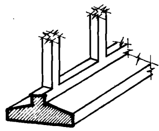
H.2.4. d MÓNG BĂNG DƯỚI CỘT
