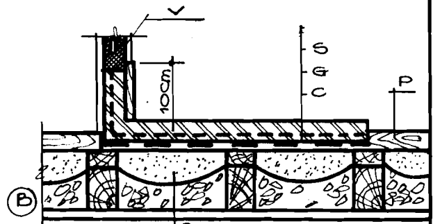
H 4 - 42 b CHI TIẾT CHỐNG THÂM SÀN GỖ
