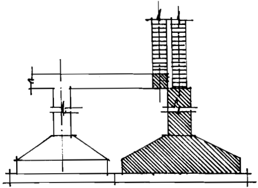
MÓNG Ở KHÊ LÙN . (KIỂU CÔNG SƠN)
