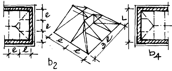
HÌNH 7-16 KẾT CẤU ĐOẠN ĐẦU HỒI KHU NÓC a1. MẶT ĐỨNG a2. MẶT BẰNG b1. KHU NÓC BÍT DỐC b1. RỒNG 2L CÓ 1 BẢN KÈO TRUNG GIẢN b3. RỒNG 4L CÓ 3 BẢN KÈO TRUNG GIẢN b4. 3l < L < 4l . c KHU NÓC CÓ KHU ĐĨẢ b2. RỒNG 3l CÓ 2 BẢN KÈO TRUNG GIẢN.
