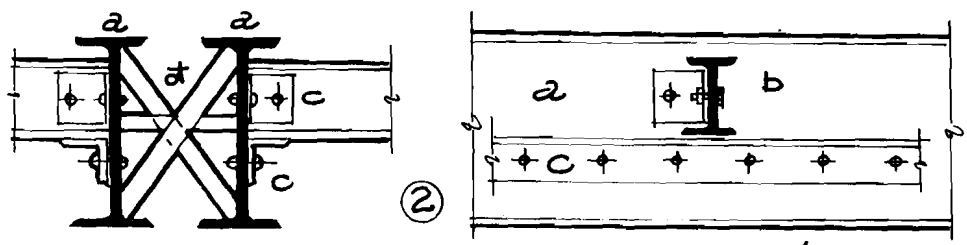
H.4.22 LIÊN KẾT DÃM PHỤ VÀO DÃM CHÍNH
