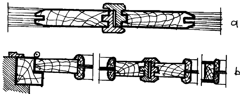
Hình 5.27 CẦU TẠO CỬA KÍNH
