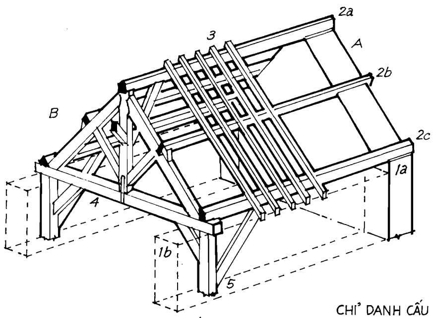
HÌNH 7-9 KẾT CẤU CHỊU LỰC A. KẾT CẤU TƯỜNG THU HỒI B. KẾT CẤU SƯỜN NÓC
