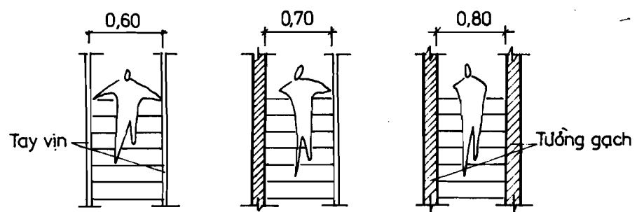
H6_6a_ Khoảng rộng cần để đón vị người đi lên xuống
