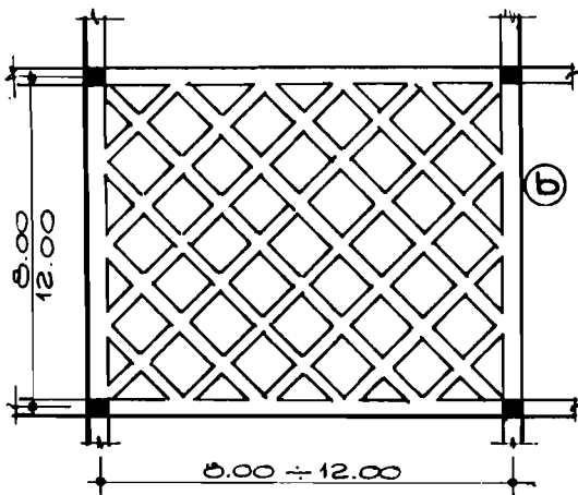
H. 4-33 SÀN Ô CỜ B.T.C.T LẮP GHEP
