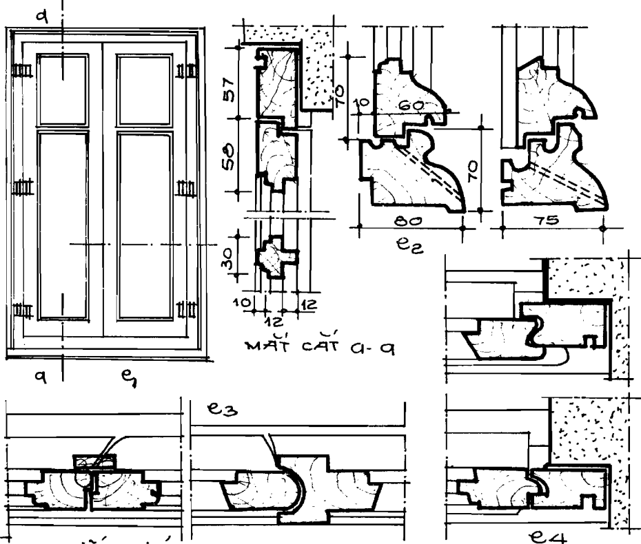
H.57D: KHE TIẾP GIÁP
