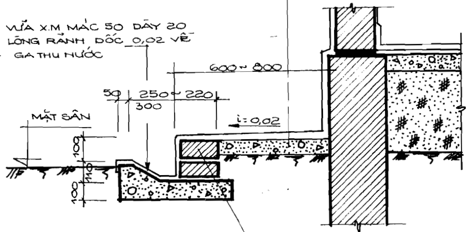
H.3.18 RÀNH THOÁT NƯỚC QUANH NHÀ
