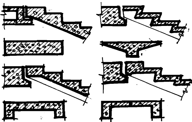
H. 36. CẦU THANG LẤP GHEP CẦU KIÊN LỚN
