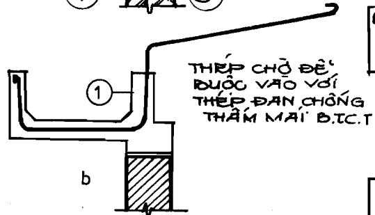
Hình 7.37B GIẰNG MĂNG NƯỚC BÊ. TÔNG CỖT THÉP
