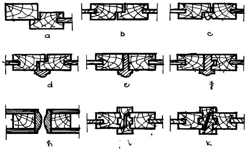
HÌNH 5-24C CHI TIẾT TIẾP GIÁP CỬA & CÁN H CỬA
