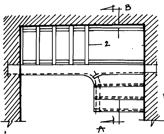
HÌNH 6-18 GHEP NỐI DẪM THANG
