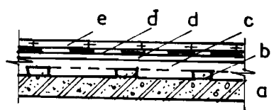
H4.54 a - Mặt sàn ván gỗ lát trên ván thô
