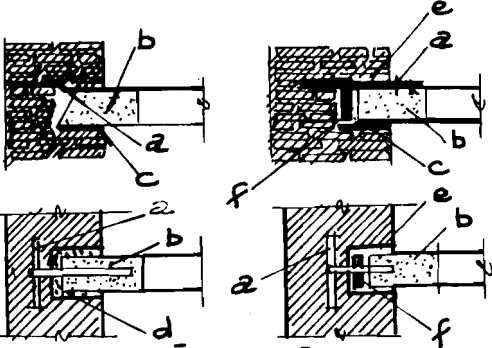
TƯỜNG DÂY 2 GẠCH
