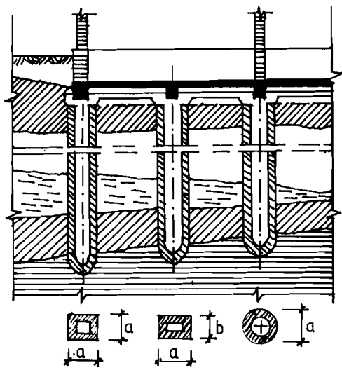
H.2.9.a MÓNG GIẾNG CHÌM (TRỤ CHÌẾC)
