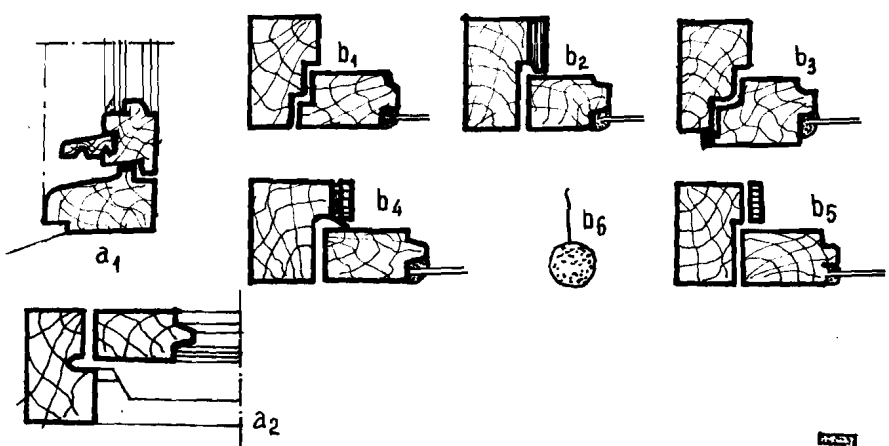
HÌNH 5.7F. CHI TIẾT CẤU TẠO NGĂN GIÓ LƯA Ở KHẸ CỬA BỐ
