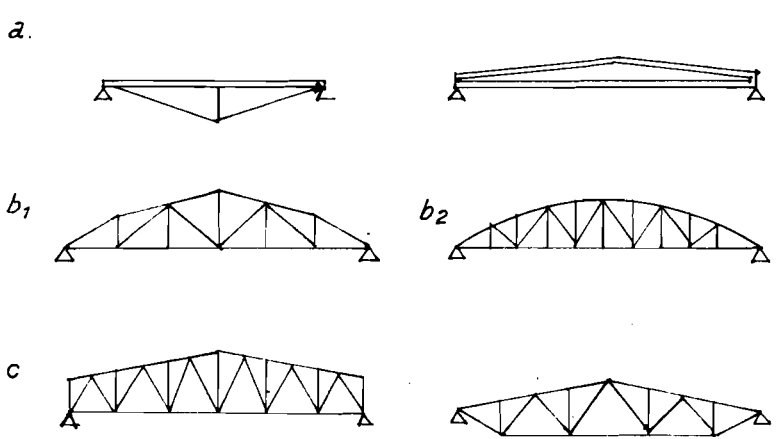
HÌNH 7.10A. CÁC DẠNG SƯỜN NÓC a. DẪM b 1 . DẪN ĐA GIÁC, b 2 DẪN CUNG TRÒN c. DẪN HÌNH THANG.
