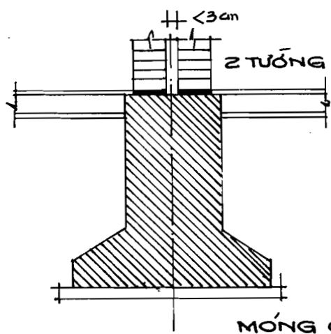
HÌNH 2-14 MÓNG Ở KHÊ BIẾN DẠNG
