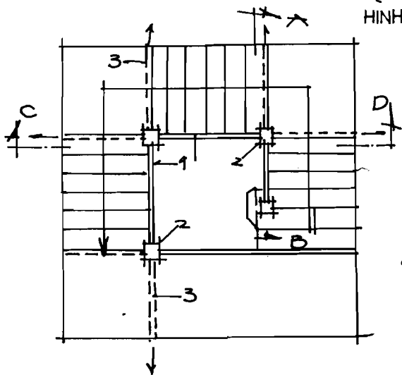
HÌNH 6-19b CẤU TẠO CHIỀU NGHI' GIẢI PHÁP DẦM THANG VÃ TRỤ ĐƯU TRUNG GIÀN.
