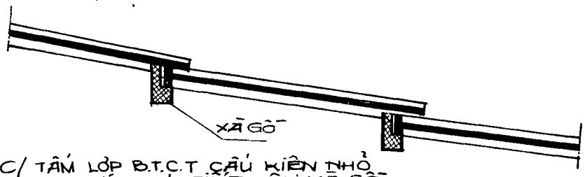
MÁI PHÂN CÁCH ĐẲNG Đ.T.C.T LẮP GHEP LOẠI MÁI DỐC VÀ MÁI ĐẲNG
