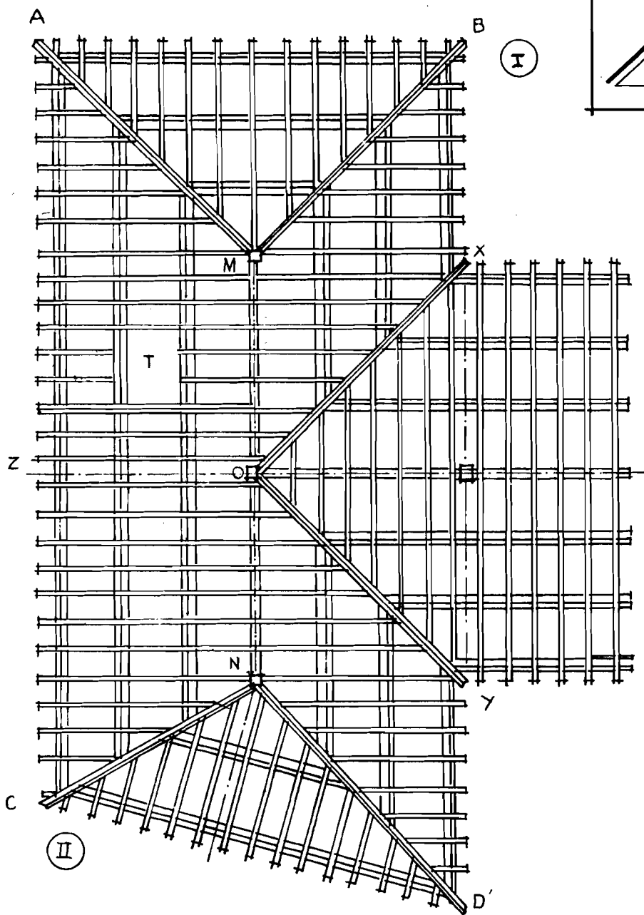
HÌNH 7.20 KHU NỐC VÀ MẠNG XÓI (RANH MÁI)
