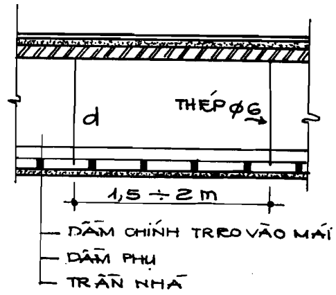
CẤU TẠO MÁI BẰNG CÁCH NHIỆT
