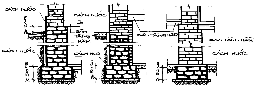
H.2.3. CẤU TẠO MÓNG XÂY ĐÁ HỘC
