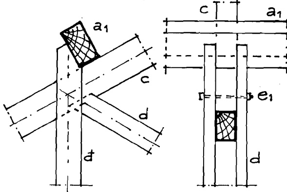
HÌNH 7.12C: LIÊN KẾT MẶT TRUNG GIAN.
