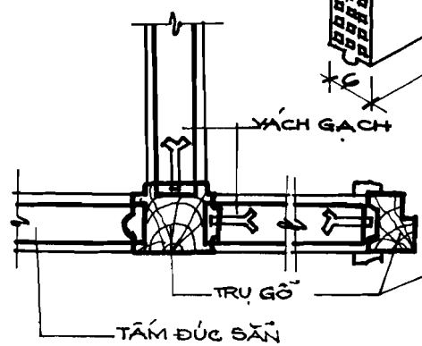
H3.28 TƯỜNG NGĂN BẰNG GẠCH
