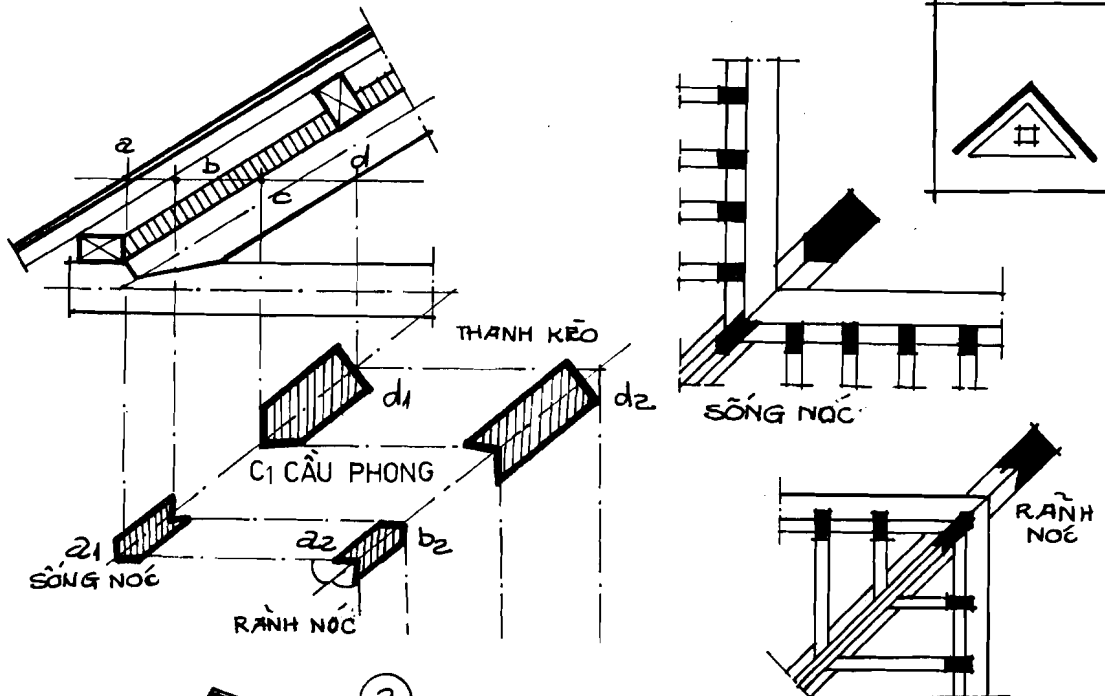
H 7-212 KHU NÓC TIẾT DIỆN NGANG CẦU PHONG VÀ THANH KÈO CHỊU MĂNG XÔI VÀ GỖ SÔNG NÓC
