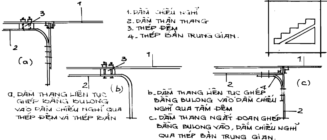
H6.25 LIÊN KẾT DÂY THANG VÀO DÂY CHÌU NGHĨ
