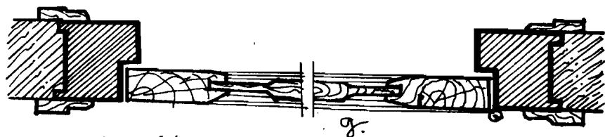
Hình 5.26B MẶT CẮT NGANG CỦA MỘT CỬA PANO.
