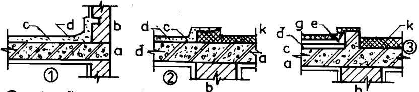
H4.47 - Mặt sàn ban công
