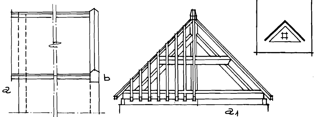
H 7-15. KẾT CẤU ĐOẠN ĐẦU HỒI NHÀ 2 MÁI a. MÁI ĐƯA RA KHỎI TƯỜNG b. TƯỜNG CHE MÁI
