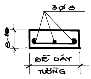
H3.8 GIĂNG TƯỜNG
