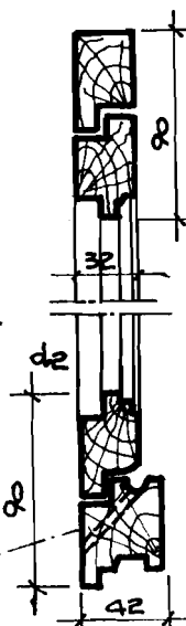
HÌNH 5.10D CỬA SỔ LẬT
