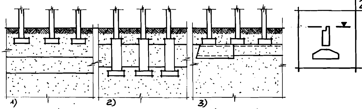
Hình 2.5a CÁC LOẠI MÓNG NHÀ TƯỜNG KHỐI KHI ĐẤT CHẶT VÀ TÍNH NỀN LƯN NHỎ. 1,2) MÓNG BẰNG KHI TẢI TRỌNG NHỎ & TRUNG BÌNH 3) MÓNG ĐẼ BẰNG B.T.C.T KHI TẢI TRỌNG LỚN
