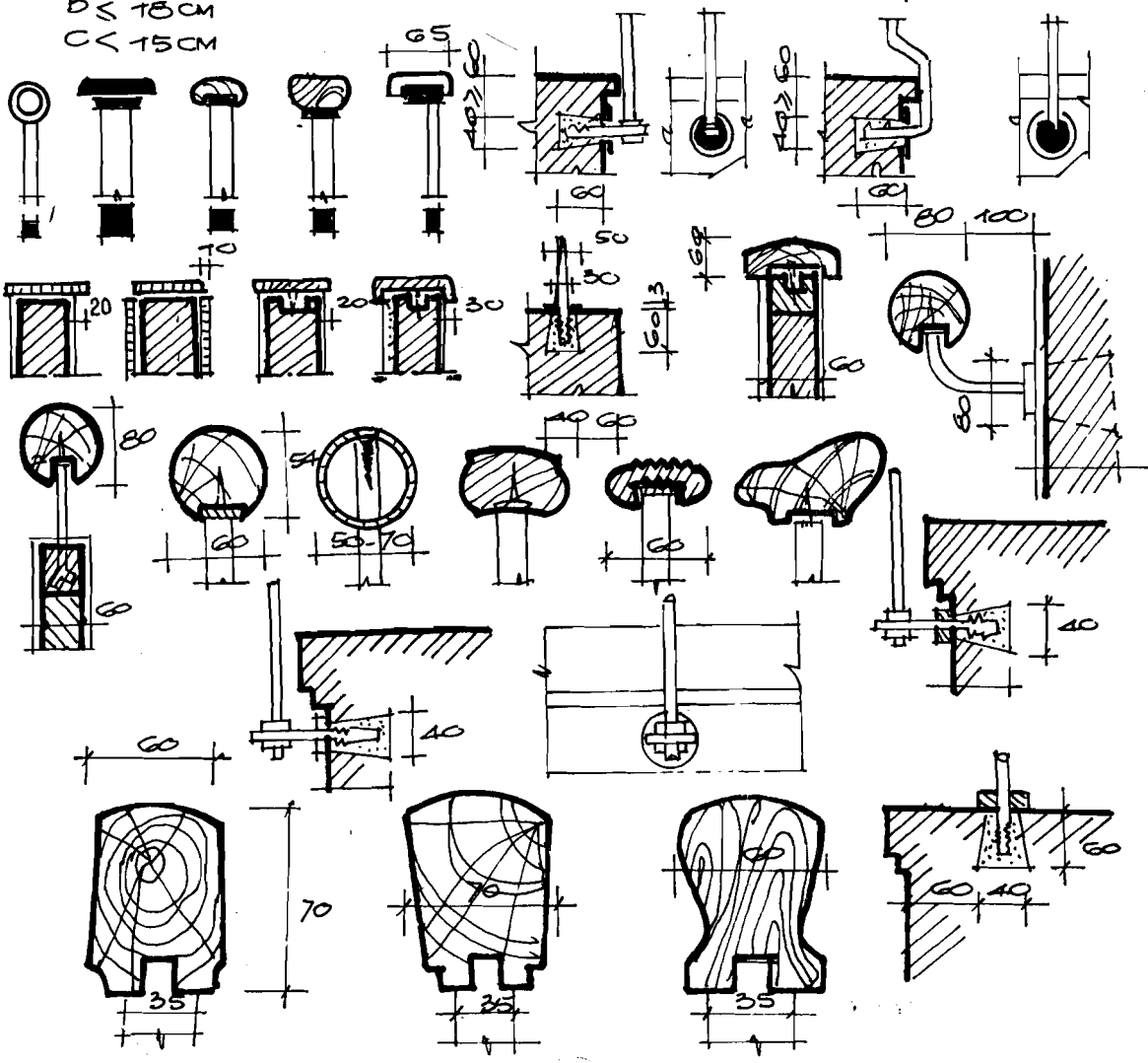
HINH 6 - 38 LAN CAN - TAY VIN
