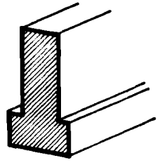
H.2.4. c MÓNG BĂNG DƯỚI TƯỜNG
