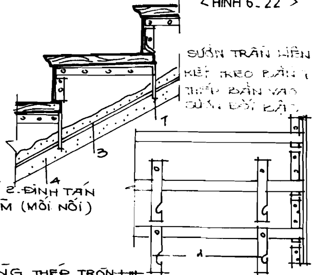
SƯỜN TRẦN LIÊN KẾT TREO BẰNG THÉP TRÒN HOẶC THÉP ĐÀN VÀO SƯỜN ĐẮC THANG
