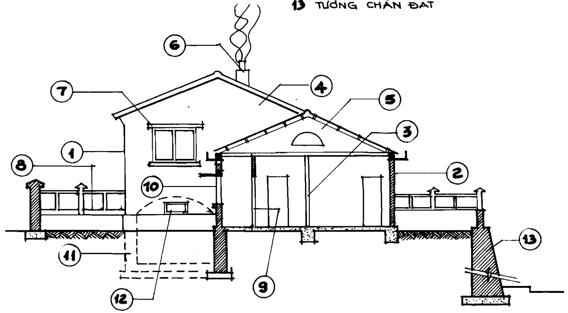
H3.1 MẶT ĐẤT TƯỜNG RÀO
