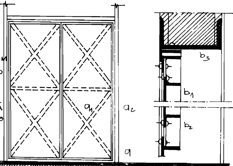
H.5.31 CỬA BẰNG KÍNH - CHẤT Dẻo - CHI TIẾT HẦM ỔN ĐỊNH
