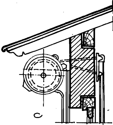
Hình 5.34a CỬA CUỐN a- CÁC LOẠI CỬA CUỐN b- MẶT CẮT DỌC MỘT CỬA CUỐN b 1 - DẠNG CỬA CUỐN MINH HỌA CHO MẶT CẮT b 2 - MẶT CẮT DỌC MỘT TẦM CỬA CUỐN c- CHI TIẾT BỘ PHẦN CUỐN CỬA d- MẶT CẮT NGANG CỬA CUỐN
