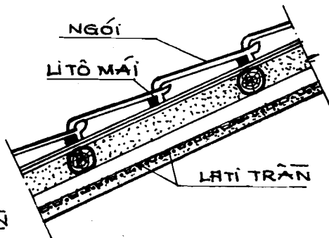
Hình 7.41 A. TRẦN ÁP MÁI 2. TRẦN ÁP MÁI B.C MẶT CẮT. CHI TIẾT
