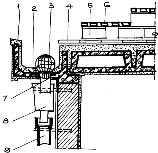
CẤU TẠO MIẾNG THU NƯỚC B.T.C.T LẤP GHEP
