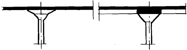
H.4.30: SÀN NẴM CÁC LOẠI ĐẦU CỘT
