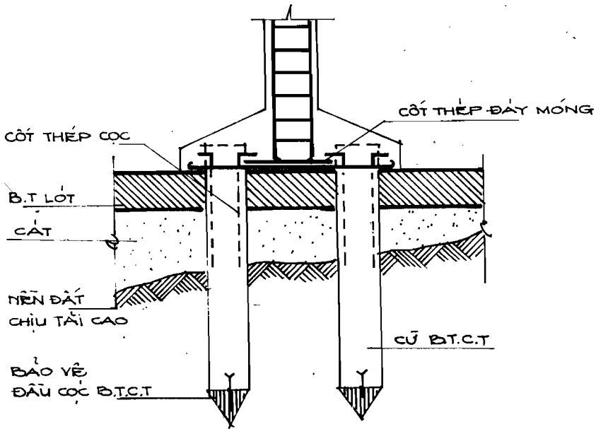
H.2.10 MÓNG TRÊN CỌC B.T.C.T (LIÊN KẾT GIỮA CỤ VÀ KHỐI MÓNG)
