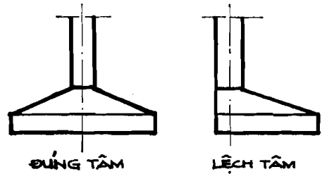
H.2.4. MÓNG THEO HÌNH THỨC CHỊU LỰC
