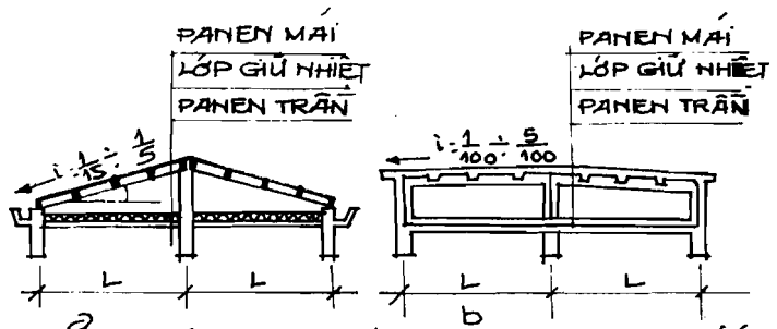
MÁI PHÂN CÁCH ĐẲNG Đ.T.C.T LẮP GHEP LOẠI MÁI DỐC VÀ MÁI ĐẲNG
