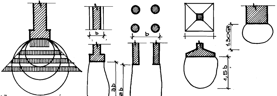
HÌNH 2.2b SƠ ĐỒ SỨC CHỊU NỀN CÁN BẦU CỦA ĐẤT NỀN DO TÁC ĐỘNG CỦA MÓNG NHÀ
