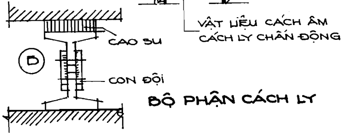
Hình 2.13a MÓNG CHỊU TẢI TRỌNG ĐỘNG (CHÂN ĐỘNG TỬ ĐÊN TRONG CÔNG TRÌNH)
