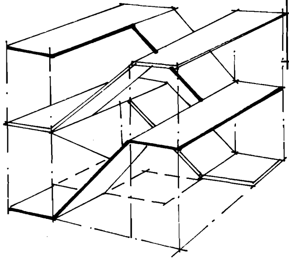
HG. 41a. GIẢI PHÁP THIẾT KẾ CẦU THANG ĐÁP ỨNG YÊU CẦU LƯU LƯỢNG NGƯỜI ĐI LẠI CAO MÃ KHÔNG CẦN TĂNG THÊM DIỆN TÍCH CỦA BUỒNG THANG.
