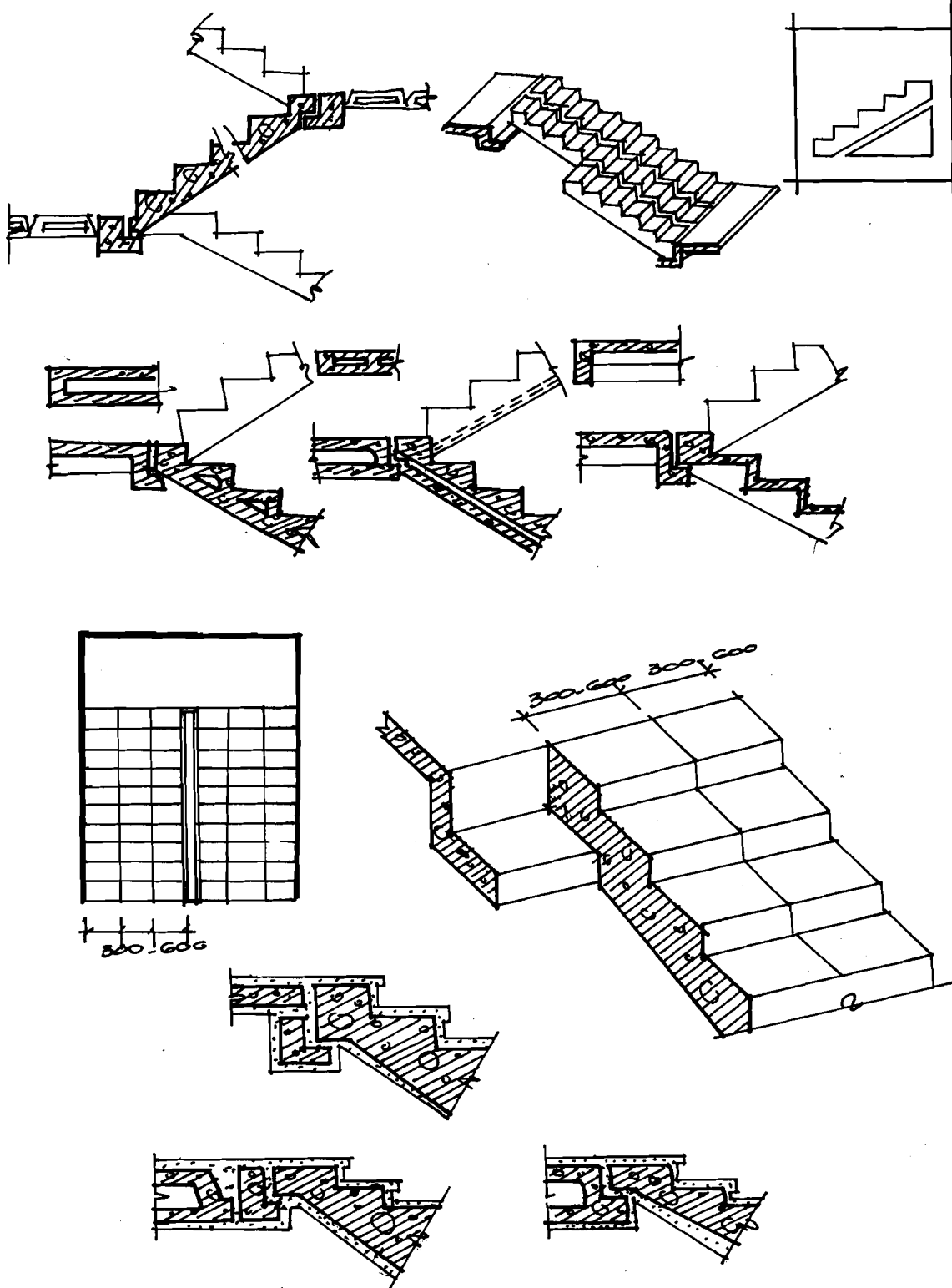
Hình 6.35 CẦU THANG LẮP GHÉP CẦU KIẾN TRUNG BÌNH
