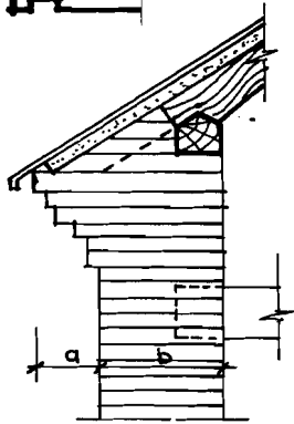
MÁI ĐUA KHI a \leq b/2
