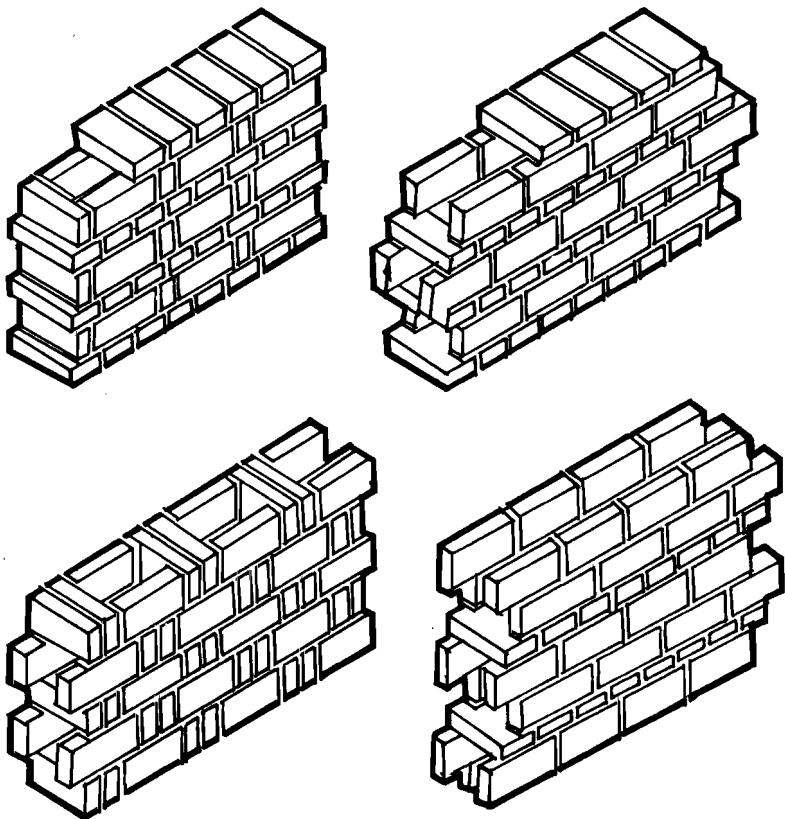
HÌNH 3.25 TƯỜNG GẠCH NHIỆT : TƯỜNG RỖNG
