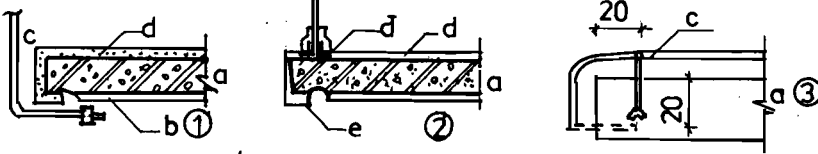
H4.46b - Chi tiết cấu tạo lan can thoáng tại ban công
