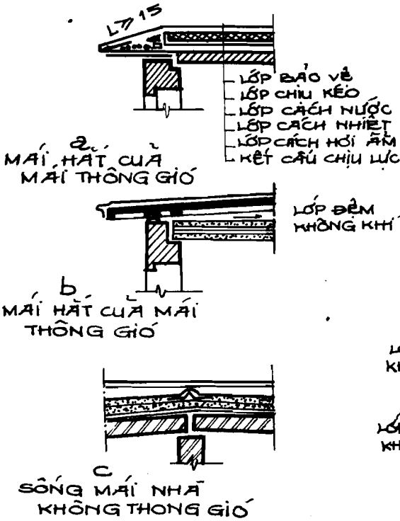
Hình 7.32 CẤU TẠO MÁI BẰNG
