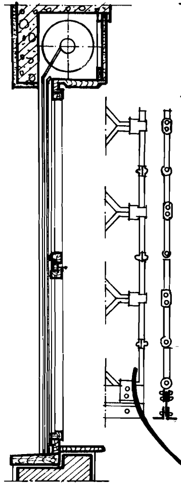
Hình 5.34a CỬA CUỐN a- CÁC LOẠI CỬA CUỐN b- MẶT CẮT DỌC MỘT CỬA CUỐN b 1 - DẠNG CỬA CUỐN MINH HỌA CHO MẶT CẮT b 2 - MẶT CẮT DỌC MỘT TẦM CỬA CUỐN c- CHI TIẾT BỘ PHẦN CUỐN CỬA d- MẶT CẮT NGANG CỬA CUỐN
