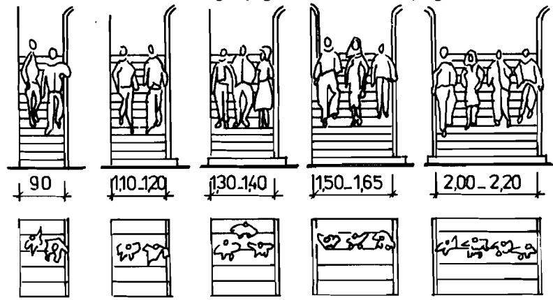
H6_6a_ Khoảng rộng cần để đón vị người đi lên xuống
