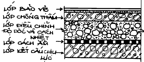
CẤU TẠO MÁI BẰNG CÁCH NHIỆT
