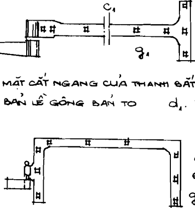
g 2 . THANH SẮT GIỮ CỬA Ở BÀN LỀ GÔNG DÙNG CHO CHIẾ
