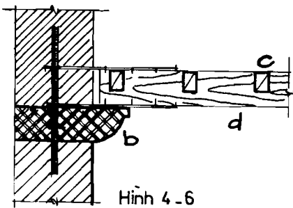
DÂM GÁC LÊN TƯỜNG
