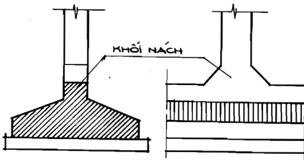
H.2.8a MÓNG BĂNG DƯỚI CỘT
