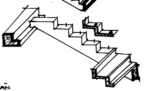
H. 37a. LIÊN KẾT GIỮA CÁC CẦU KIÊN LIÊN KẾT BẰNG CHỐT
