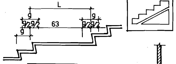
H6.8_Tham số cấu tạo chiếu nghỉ
