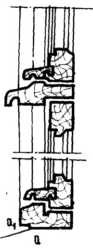
HÌNH 5.8 CẤU TẠO GỖ HẠT NƯỚC
