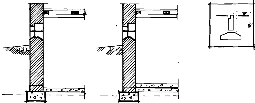
HÌNH 2-18a MỨC NƯỚC NGẦM Ở DƯỚI MẶT NỀN TẦNG HẦM
