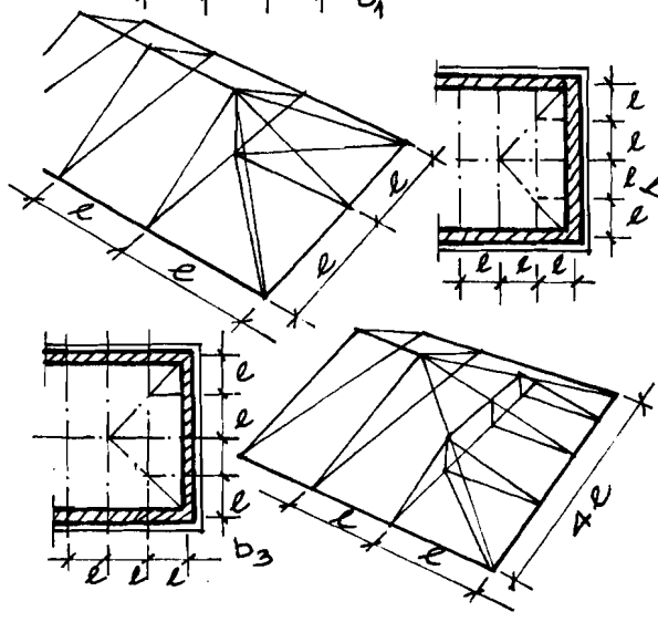
HÌNH 7-16 KẾT CẤU ĐOẠN ĐẦU HỒI KHU NÓC a1. MẶT ĐỨNG a2. MẶT BẰNG b1. KHU NÓC BÍT DỐC b1. RỒNG 2L CÓ 1 BẢN KÈO TRUNG GIẢN b3. RỒNG 4L CÓ 3 BẢN KÈO TRUNG GIẢN b4. 3l < L < 4l . c KHU NÓC CÓ KHU ĐĨẢ b2. RỒNG 3l CÓ 2 BẢN KÈO TRUNG GIẢN.
