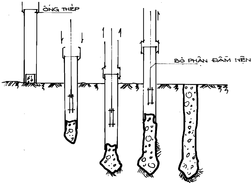
H.2.11 CỌC NHỒI
