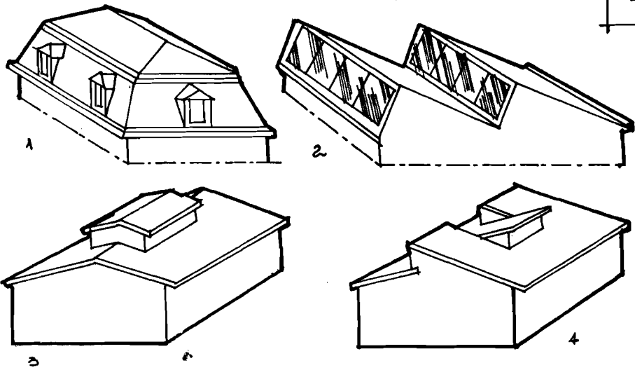
HÌNH 7-6B - HÌNH THỨC MÁI ĐỐC
