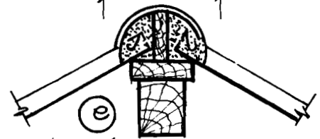
d, e. CHI TIẾT ĐÌNH MÁI BẰNG FIBRÔ-XI-MĂNG VÀ MŨ NGÔI
