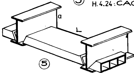
③ H.4.24: CÁC KIỂU TRẦN CỘ ĐIỆN ④
