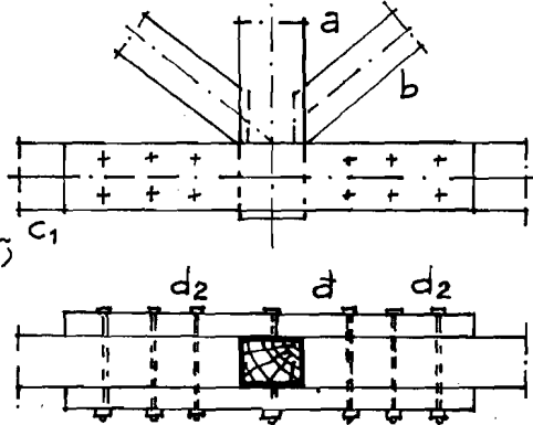
HÌNH 7.12B. LIÊN KẾT MẶT GIỮA
