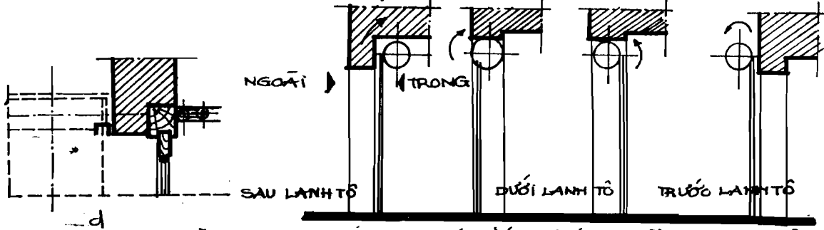
Hình 5.34b SƠ ĐỒ VỊ TRÍ SẮT HƯỚNG DẪN VÀ BỘ PHẦN CUỐN
