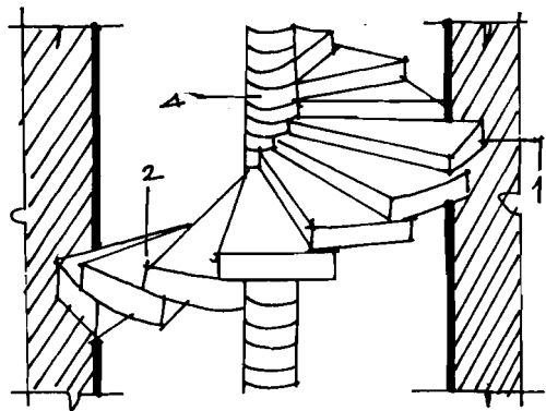
CẦU THANG CÓ BẬC THANG MỘT KHỐI CHỖNG LÊN NHAU
