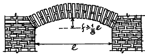
H.3.2b LANHTÔ GẠCH CUỘN VỒM ( l < 2m )
