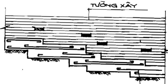
H2.6a MÓNG BẰNG DƯỚI TƯỜNG
