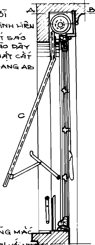
Hình 5.18A CỬA SẠO CUỐN
