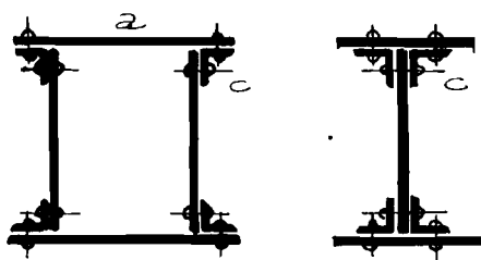
H.4.20: GHEP DÂM THÉP BẢN
