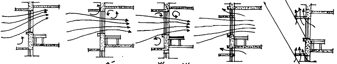
H3.12 TẮM CHE CHẮN NẮNG
