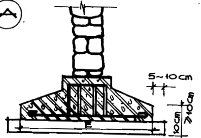
MÓNG CHIẾC DƯỚI CỘT
