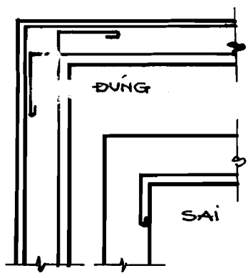
GHI TIẾT ĐẶT CỘT THÉP TRONG GIĂNG TƯỜNG B.T.C.T.
