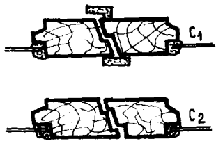
HÌNH 5.7F. CHI TIẾT CẤU TẠO NGĂN GIÓ LƯA Ở KHẸ CỬA BỐ
