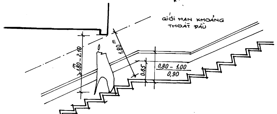
Hình 6-4 CHIỀU NGHỈ
