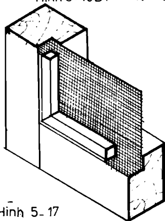
CẤU TẠO CỬA LƯỚI CHỐNG MUỖ
