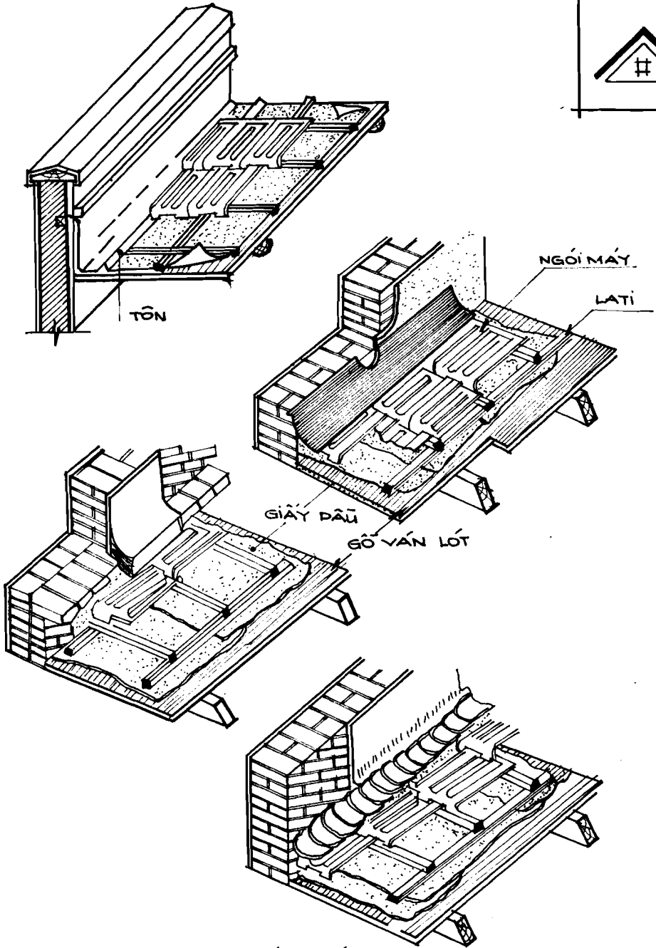
H 7.31 ; TƯỜNG CHE MÁI NGÓI
