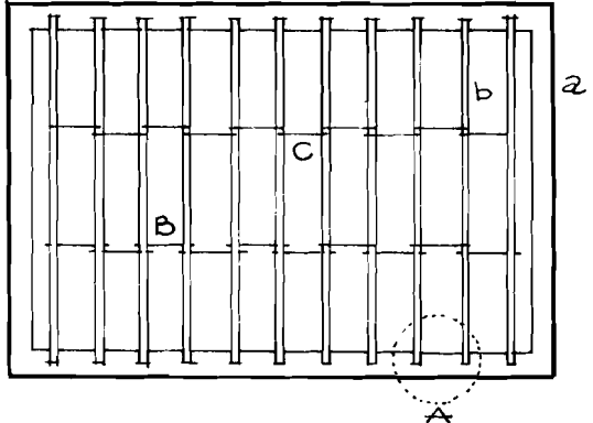
H.4.18: SƠ ĐỒ BỐ TRÍ DÂY SÀN SẮT THÉP
