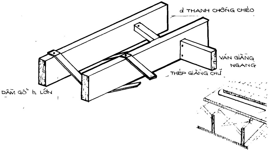
Hình 4-9 : ỔN ĐỊNH CHÔNG, LÁT DÂM a- SẮT NEO VÀO TƯỜNG b- DÂM GỖI DỌC TƯỜNG c- DÂM GỖ d- THANH GỖ CHÔNG CHÉO ĐỂ ỔN ĐỊNH DÂM SÀN
