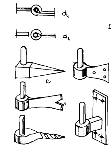
HÌNH 5.38 CÁC LOẠI BÀN LỀ GÔNG
