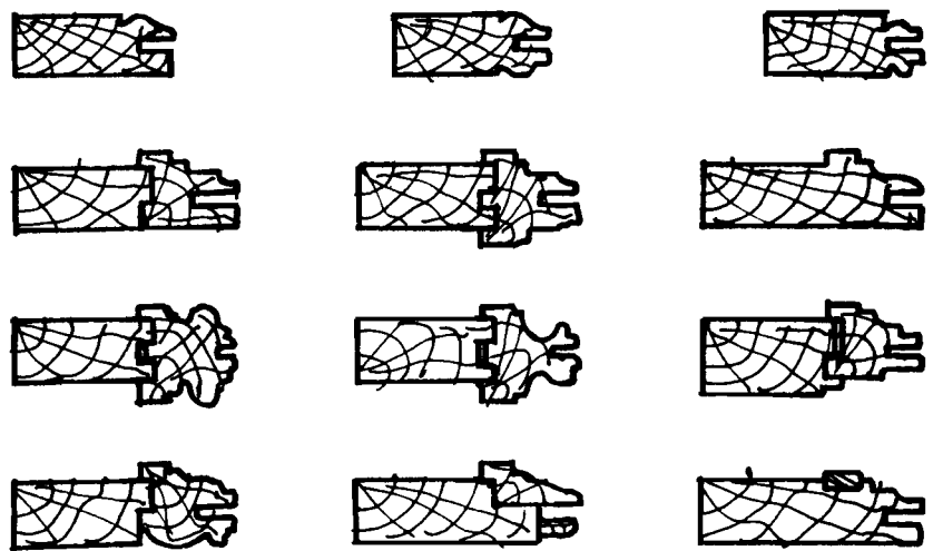
HÌNH 5-24B MẶT CẮT CÁC LOẠI KHUNG CỬA ĐI
