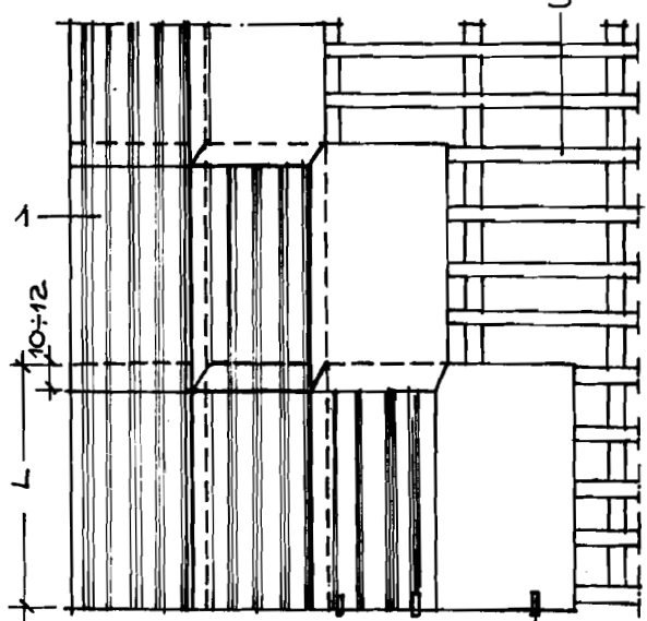
b. MẶT BẰNG LỢP MÁI CÓ CẮT GÓC 1 TẦM LỚP. 2 MÓC ĐỖ. 3 XÃ GỖ
