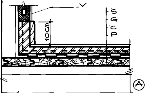
H 4 - 42 b CHI TIẾT CHỐNG THÂM SÀN GỖ
