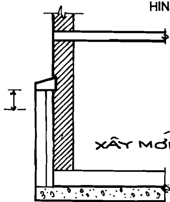
HÌNH 2-18 GIẢI PHÁP CHỐNG THÂM TẦNG HẦM
