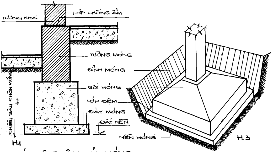
CÁC BỘ PHẬN CỦA MÓNG
