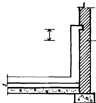
HÌNH 2-18 GIẢI PHÁP CHỐNG THÂM TẦNG HẦM
