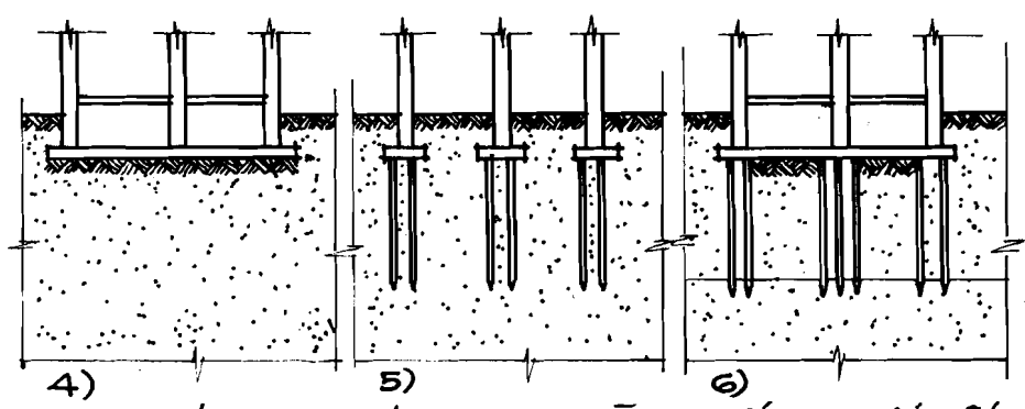
Hình 2.5b CÁC LOẠI MÓNG NHÀ TƯỜNG KHỐI KHI ĐẤT YẾU (RỐI) 4,5,6) KHI TẢI TRỌNG LỚN
