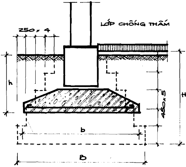
H.2.4. MÓNG THEO HÌNH THỨC CHỊU LỰC
