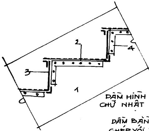
DẠM BĂNG TÔN VÀ THÉP HÌNH GHEP LẠI
