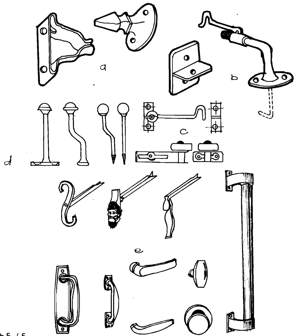
MÓC GIÓ - CHẶN CẢNH VÀ CÁC TAY NẮM CỬA
