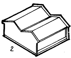
HÌNH 7.8 KẾT CẤU TƯỜNG THU HỒI CHỊU LỰC 1 MÀI HIÊN CHE TƯỜNG ĐẦU HỒI 2 TƯỜNG CHE MÀI TẠI ĐẦU HỒI
