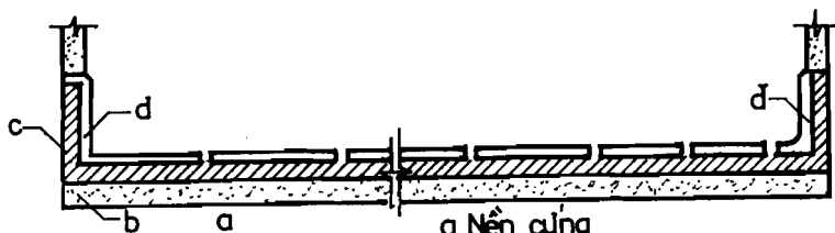
H4.55_Mặt sàn lát gạch xi măng
