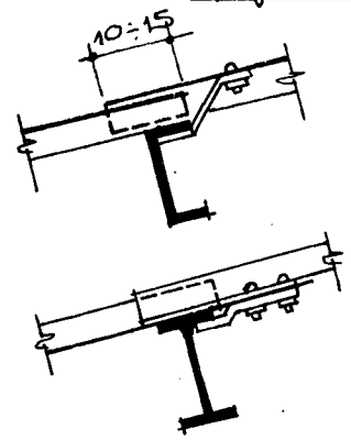
HÌNH 7-26 MÁI LỘP TÔN THIẾC TRẮNG KẼM
