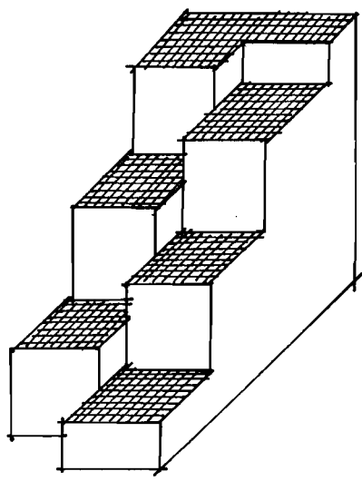
HG. 41a. GIẢI PHÁP THIẾT KẾ CẦU THANG ĐÁP ỨNG YÊU CẦU LƯU LƯỢNG NGƯỜI ĐI LẠI CAO MÃ KHÔNG CẦN TĂNG THÊM DIỆN TÍCH CỦA BUỒNG THANG.
