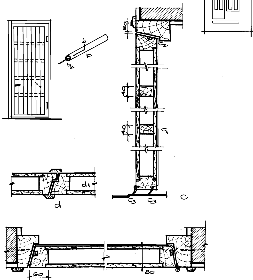
Hình 5.29 CẤU TẠO CỬA CÁCH ÂM
