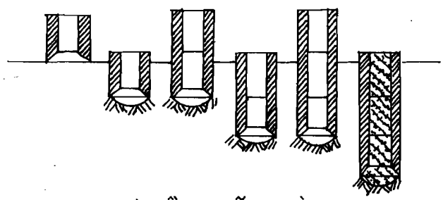
H.2.9.b SƠ ĐỒ HẠ GIẾNG CHÌM.
