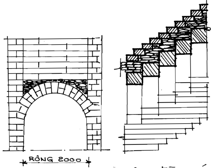
H6-30 . CẦU THANG TRONG NHÀ XÂY BẰNG ĐÁ (THÂN THANG THẰNG)
