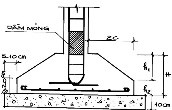
MÓNG BĂNG DƯỚI CỘT
