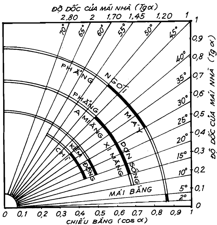
HÌNH 7-4 ĐỘ ĐỐC CỦA MÁI NHÀ THEO VẬT LIỆU LỢP
