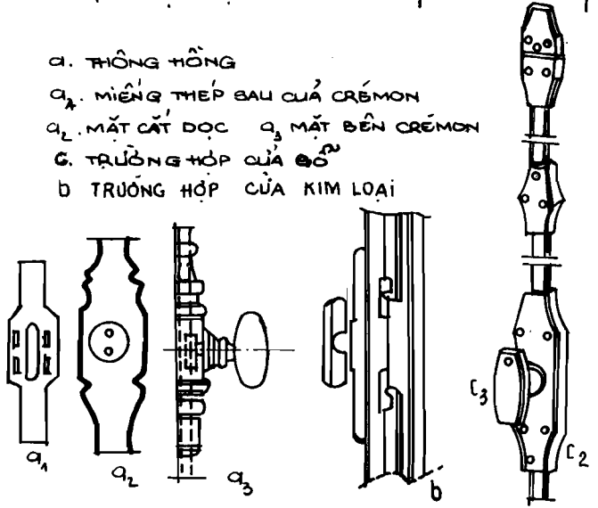
HÌNH 5.42 BỘ PHẦN THEN KHOÁ
