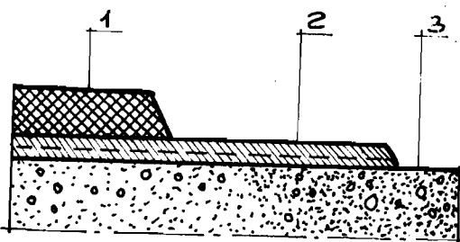
Hình 7.33c CẤU TẠO BẢO VỆ SÀN THƯỜNG
