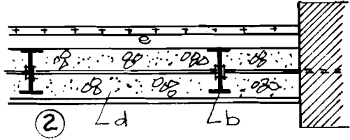
2. TƯỜNG GẠCH đ. BÊ TÔNG NHE b. DÂM THÉP e. ĐỘ GỒ c. KIỀNG SẮT g. VÁN SÀN d. SẮT GÓC h. VỮA TRÁT TRẦN l. GẠCH THÉ
