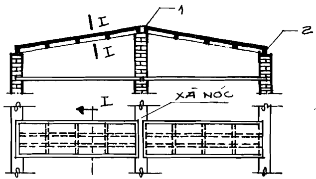
d/ TẦM LỚP PANEN ĐẶT KÊ LÊN TƯỜNG NGANG CHỊU LỰC
