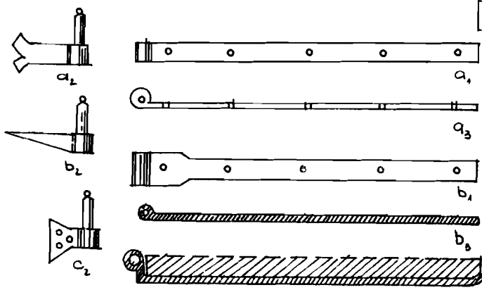
HÌNH 5.37 B. BÀN HƯỚNG DẪN LẮP ĐẶT BÀN LỀ CỬA VÀ KHOẢ
