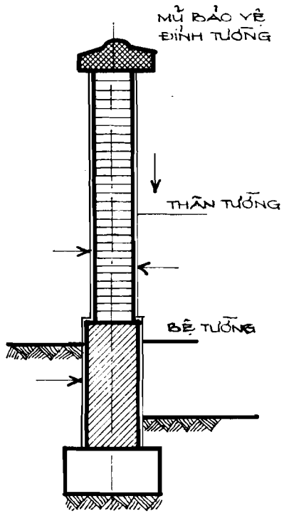
H3.1 MẶT ĐẤT TƯỜNG RÀO
