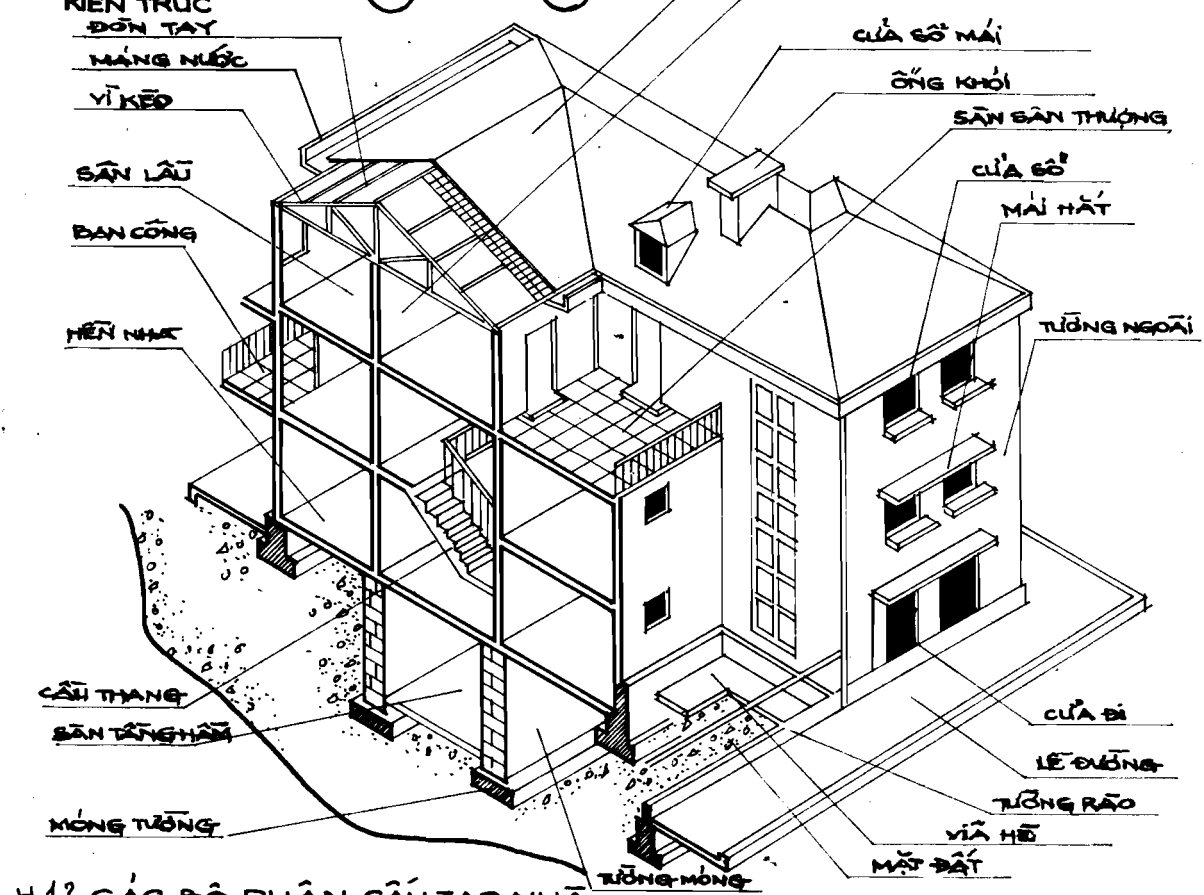
H.1.2 CÁC BỘ PHẦN CẤU TẠO NHÀ
