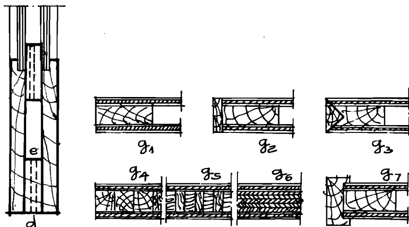
Hình 5.28B CỬA GỖ DÁN
