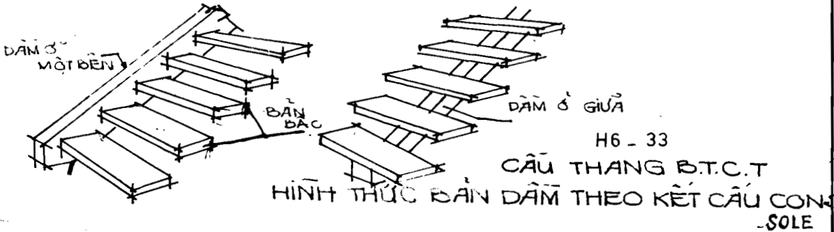
CẦU THANG B.T.C.T TOÀN KHỐI HÌNH THỨC BẢN H6-32a
