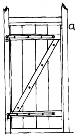
Hình 5.30B CỬA KHÔNG KHUNG
