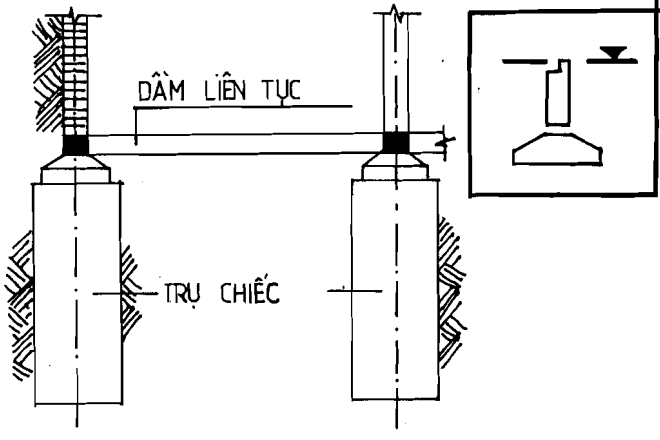
H.2.9.C MÓNG TRỤ CHÌẾC
