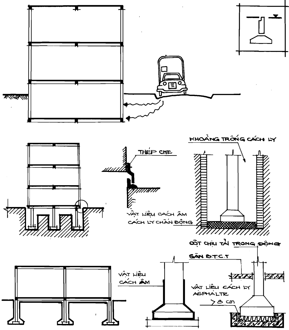
BAO QUANH MÓNG BẰNG VẬT LIỆU CÁCH ÂM
