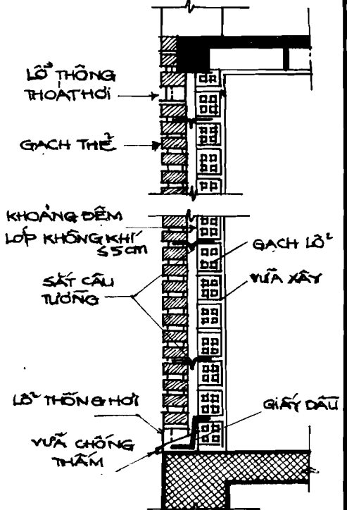
CHI TIẾT TƯỜNG GẠCH XÂY 2 LỚP CÓ KHOẢNG ĐEM KHÔNG KHÍ CÁCH NHIỆT
