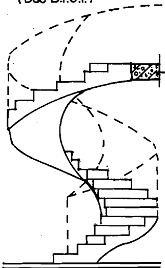
H6_40a_ Cầu thang tròn xoay trên ốc
