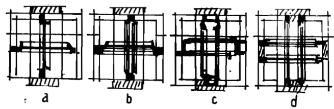
Hình.5-3 CỬA ĐỒ NHIỀU LỚP
