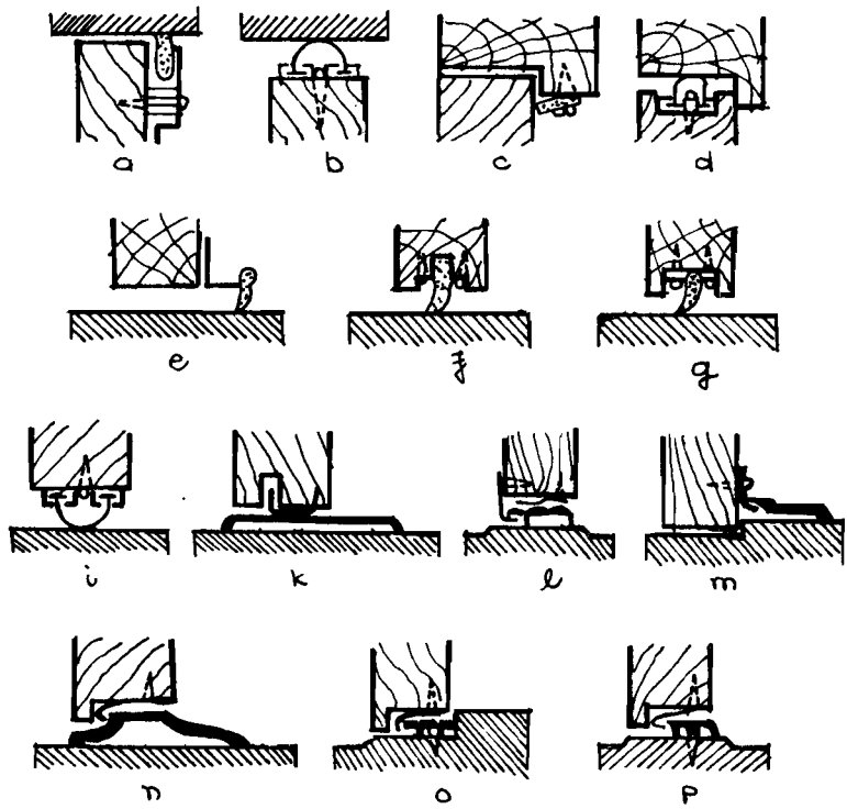
HÌNH 5.25 A CHI TIẾT CẤU TẠO CHỐNG THÂM KÍN GIÓ a, b CẤU TẠO CHO PHẦN TRÊN CỬA c, d CHỐNG THÂM, KÍN GIÓ CHO CỬA VỚI KHUNG CỬA BẰNG GỖ e, f, g CHỐNG THÂM, KÍN GIÓ CHO PHẦN DƯỚI CỬA i, k, l, m, n, o, p CẤU TẠO CHỐNG THÂM VÀ KÍN GIÓ PHẦN DƯỚI CỬA BẰNG CÁCH LIÊN KẾT VỚI NHỮNG TẦM THẾP.
