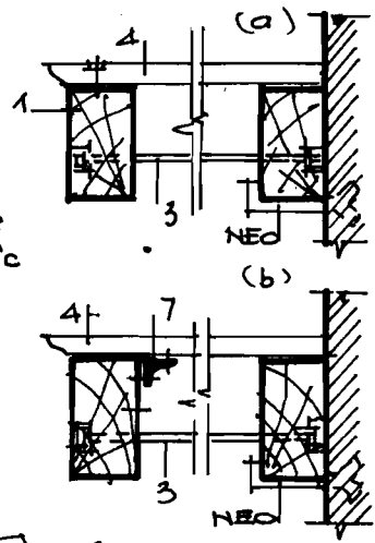
HÌNH 6-16 DẪM THANG HÌNH RĂNG CỬA HÌNH 6-17 CẤU TẠO ƠN ĐỊNH DẪM THANG (a);(b)
