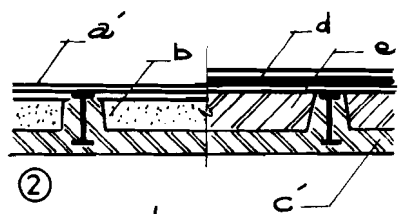
H.4.26 SÀN THÉP BÊTÔN CỐT THÉP
