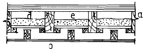
SÀN GỖ CÁCH NHIỆT - ÂM
