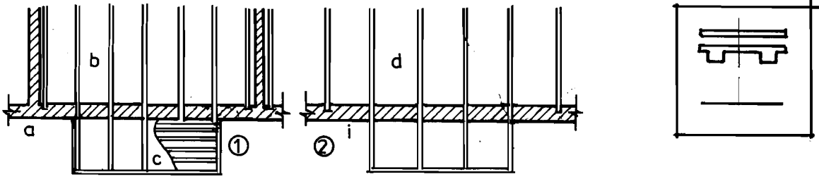
H4.46 - Kết cấu chịu lực Ban công - Lôgia
