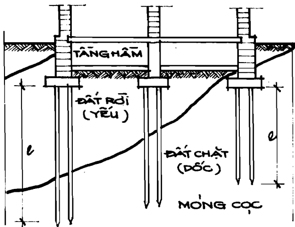
Hình 2-5e CÁC LOẠI MÔNG KHI CÁC LỚP ĐẤT NỀN CÓ CHIỀU DÀY KHÁC NHAU (GIẢI PHÁP MÔNG CỌC)
