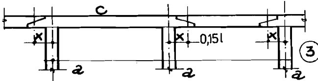
Hình 4.5: DÂM GÁC LÊN CỘT GỖ
