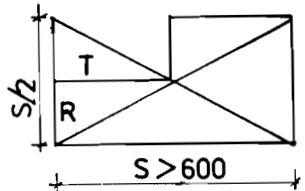
H6_6b2-Chiều rộng thang nhà công cộng
