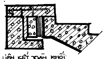
H. 37b. LIÊN KẾT GIỮA CÁC CẦU KIÊN
