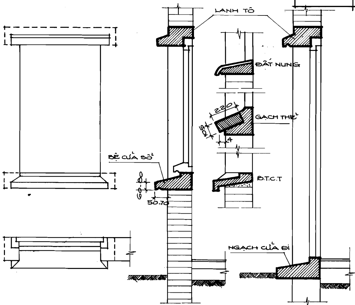
H3.11.b 1 ĐỀ CỬA BỐ
