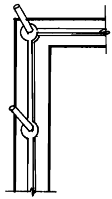
GIĂNG TƯỜNG BẰNG THÉP
