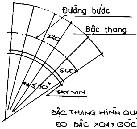
HINH 6-11 XỬ LÝ BẮC THANG
