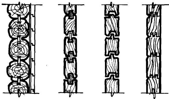
H3.30a TƯỜNG NGĂN ĐẰNG GỖ THANH GHEP
